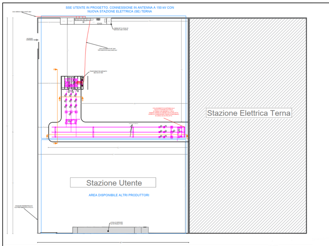
Fig. 65: Layout della Sottostazione Utente
