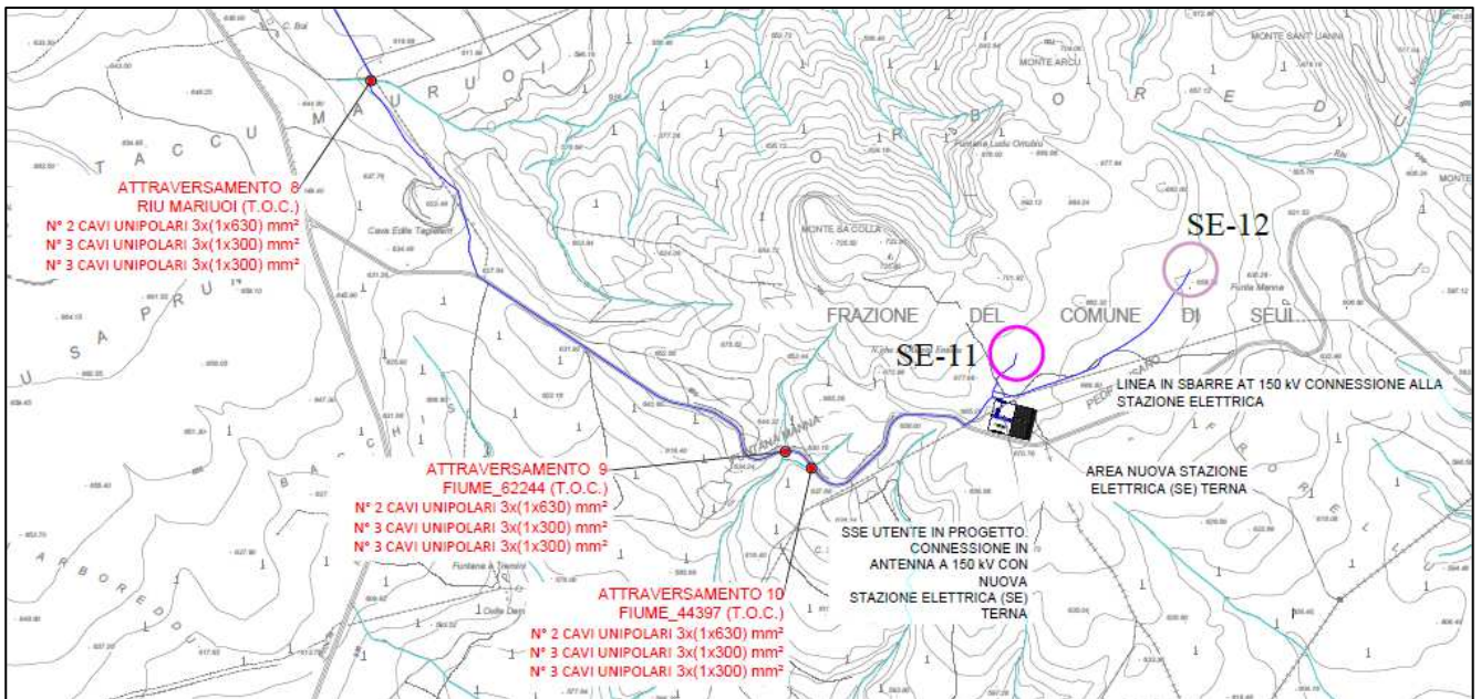
Attraversamenti corpi idrici superficiali dei cavidotti - area Sud – attraversamenti 8,9, 10 (T.O.C.)
