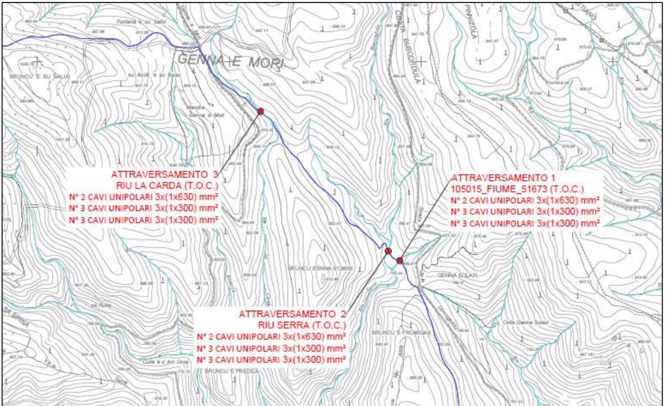
Attraversamenti corpi idrici superficiali dei cavidotti - area Nord – attraversamenti 1, 2, 3 (T.O.C.)
