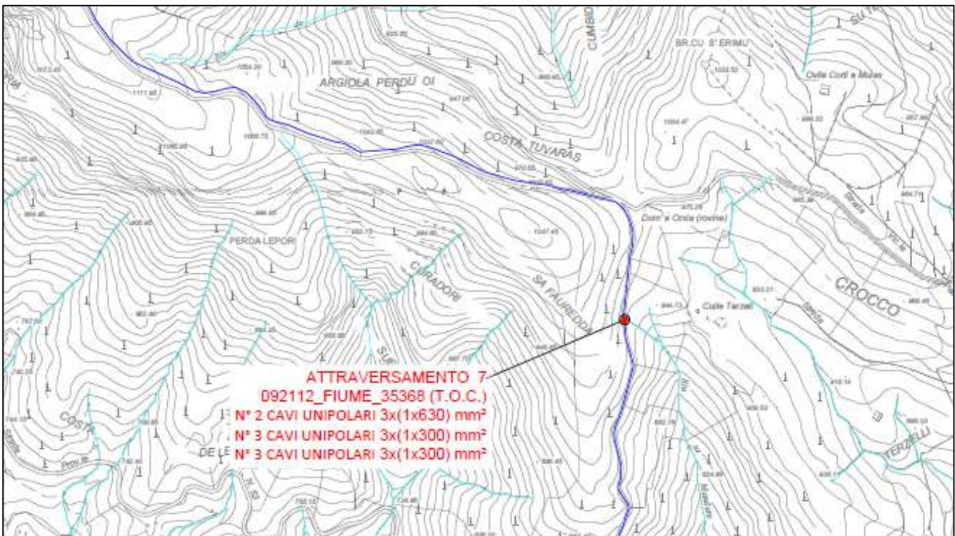
Attraversamenti corpi idrici superficiali dei cavidotti - area Nord – attraversamento 7 (T.O.C.)
