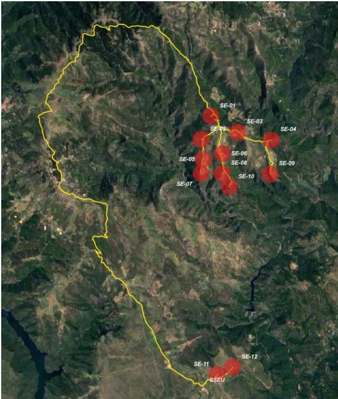
Inquadramento, layout e connessione elettrica su ortofoto – in giallo i cavidotti interrati, cerchi in tratteggio azzurro areali degli aerogeneratori (non in scala),
