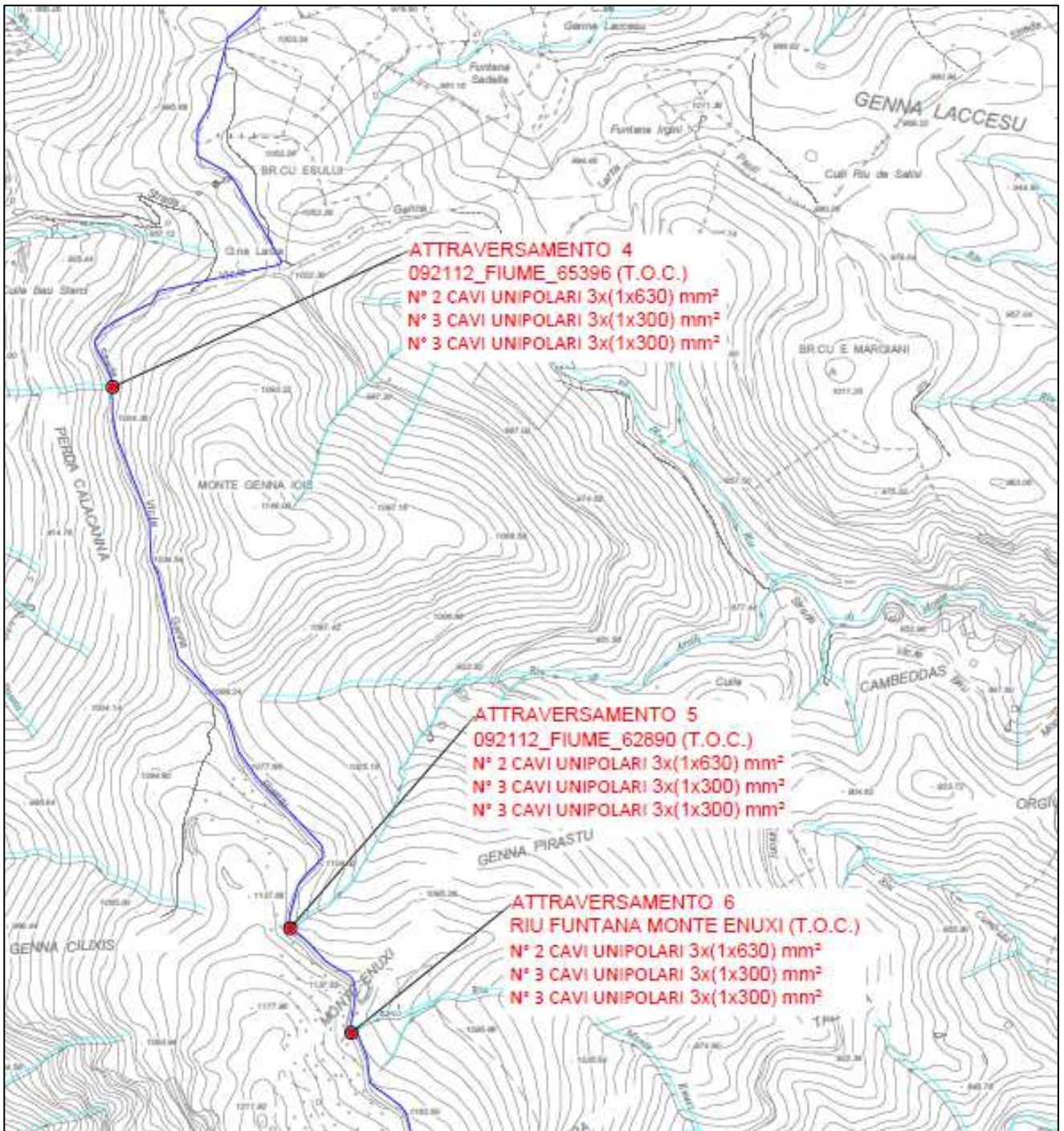
Attraversamenti corpi idrici superficiali dei cavidotti - area Nord – attraversamenti 4,5, 6 (T.O.C.)
