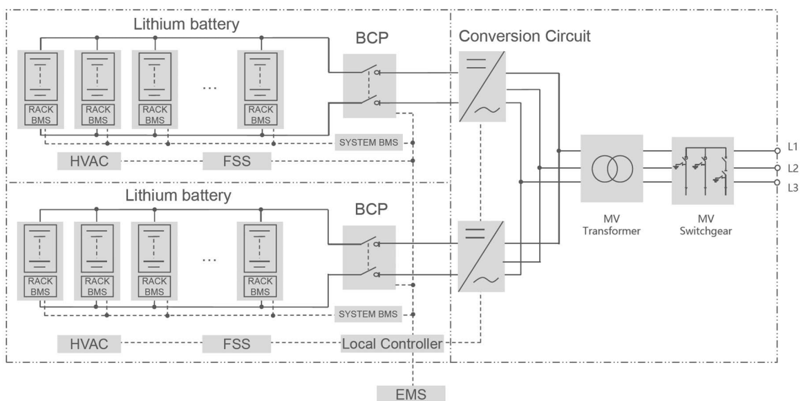
Figura 3 – Schema tipologico funzionale singolo battery block
