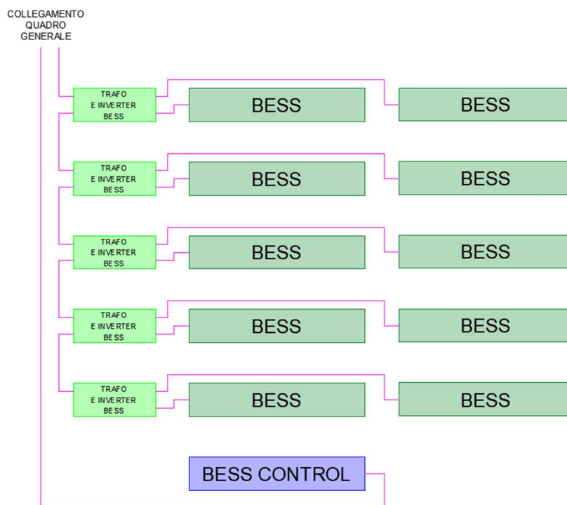
Figura 5 – Layout dell'impianto BESS all'interno dell'area disponibile.
