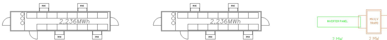
Figura 4 – Layout singolo battery block
