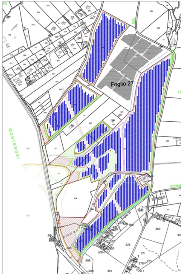
Area di progetto suddivisa in 6 sottocampi (in blu i filari di pannelli fotovoltaici; in rosso l'area testimone/controllo per il monitoraggio della produttività agricola fuori impianto, in verde le opere di mitigazione, in fucsia la recinzione, in grigio la viabilità interna).
