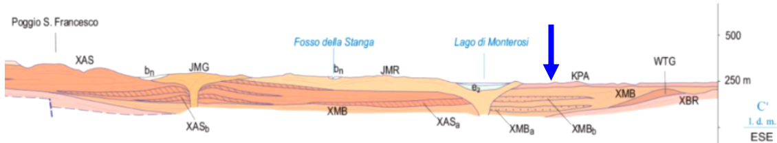
Sezione geologica d'interesse per l'area in studio
