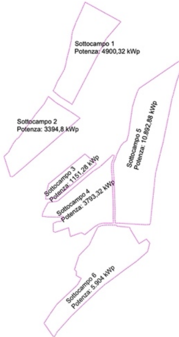
Sottocampi dell'impianto agrovoltaiico
