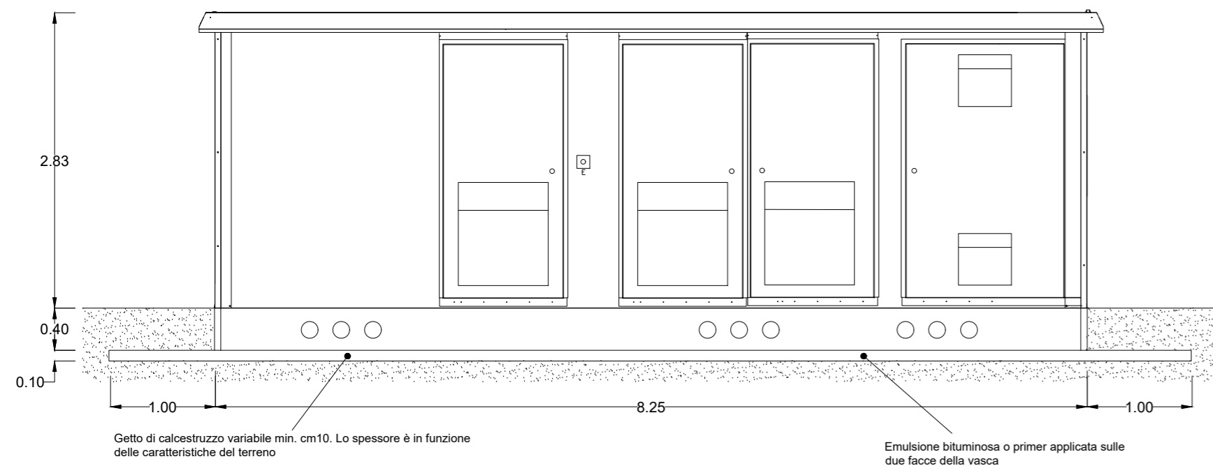
PROSPETTO FRONTALE
