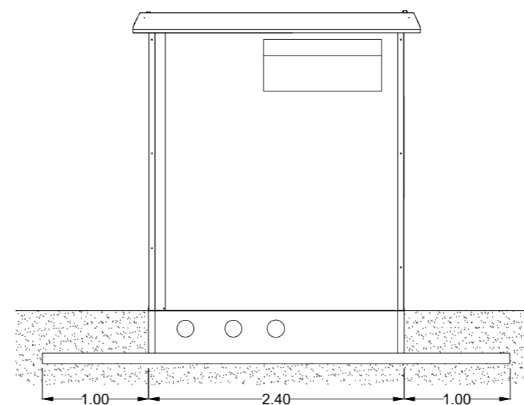
PROSPETTO LATERALE
