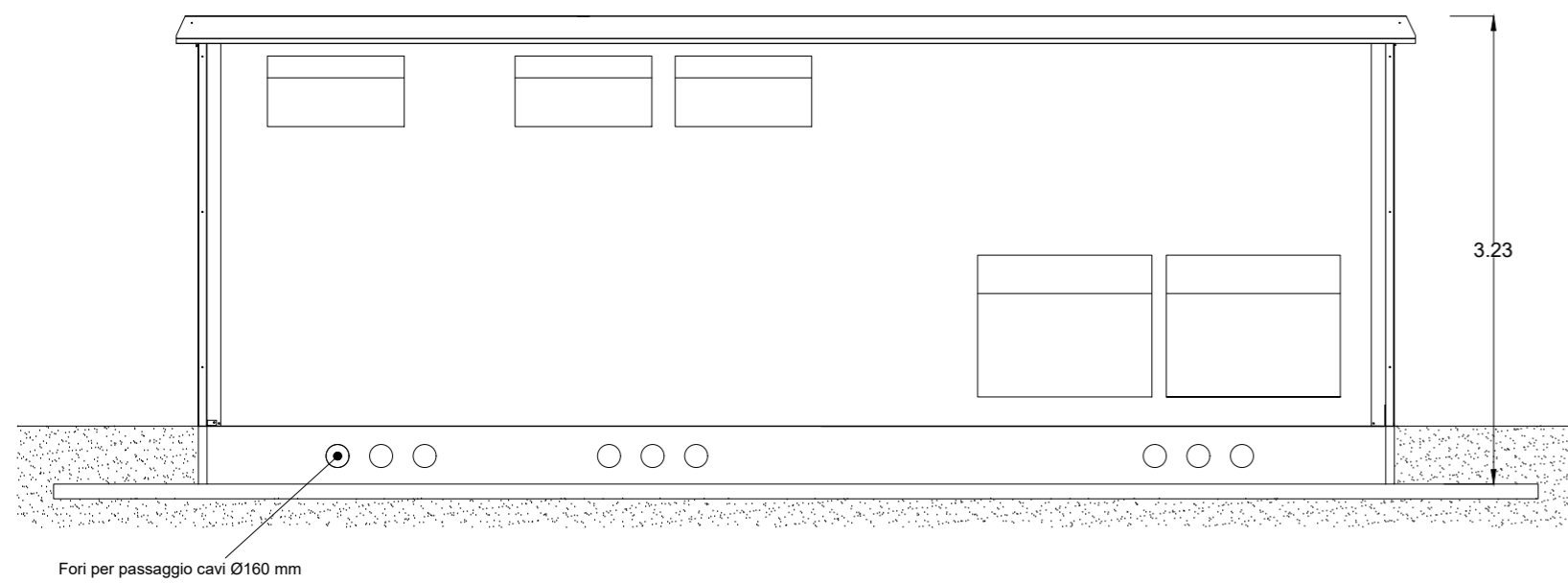
PROSPETTO FRONTALE
