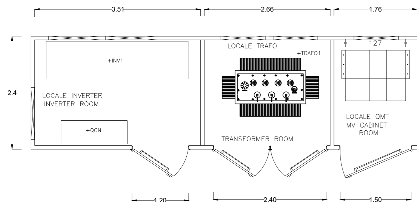
PIANTA DALL'ALTO
