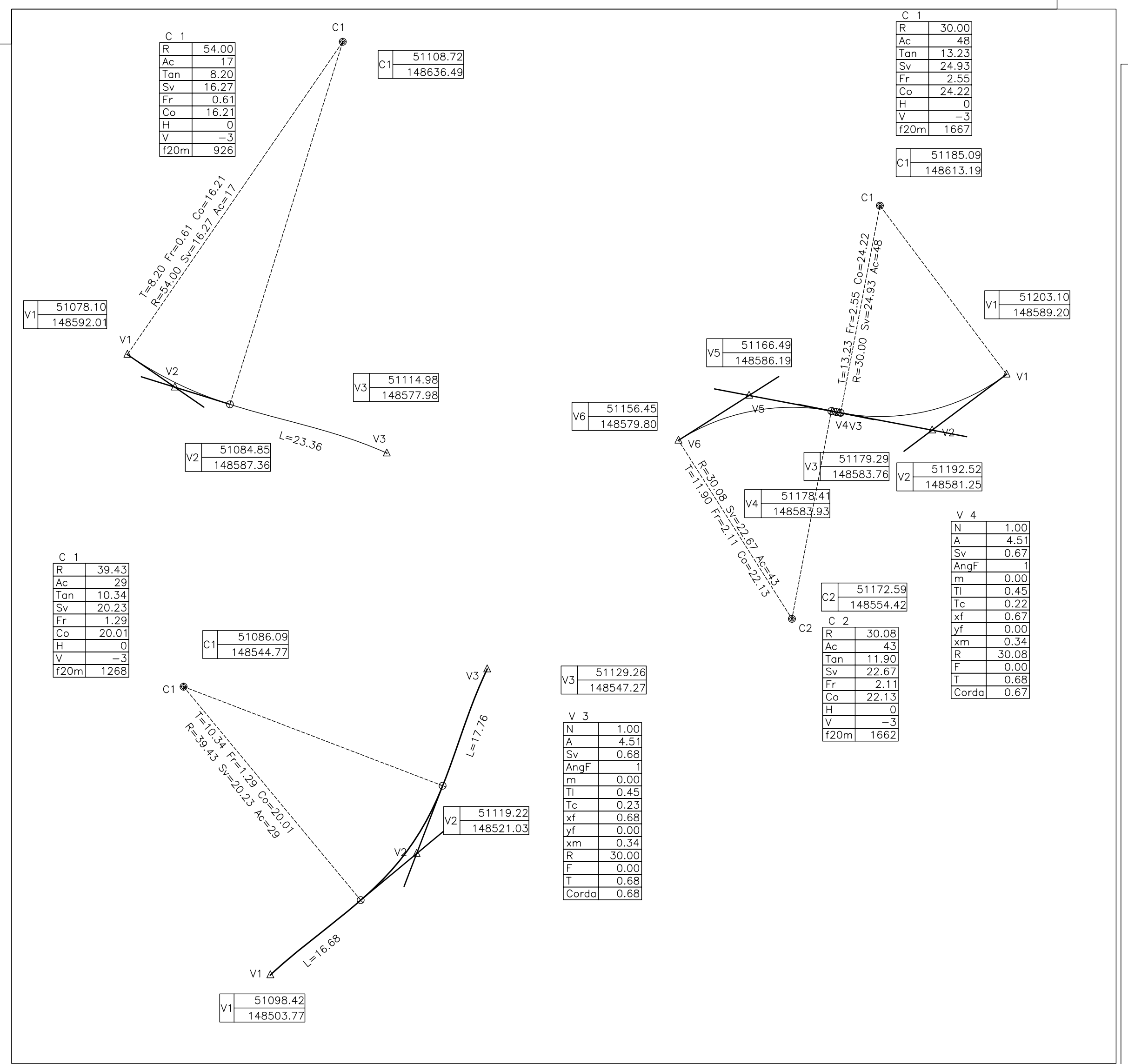
PLANIMETRIA DI TRACCIAMENTO ROTATORIA R.2 Scala 1:200
