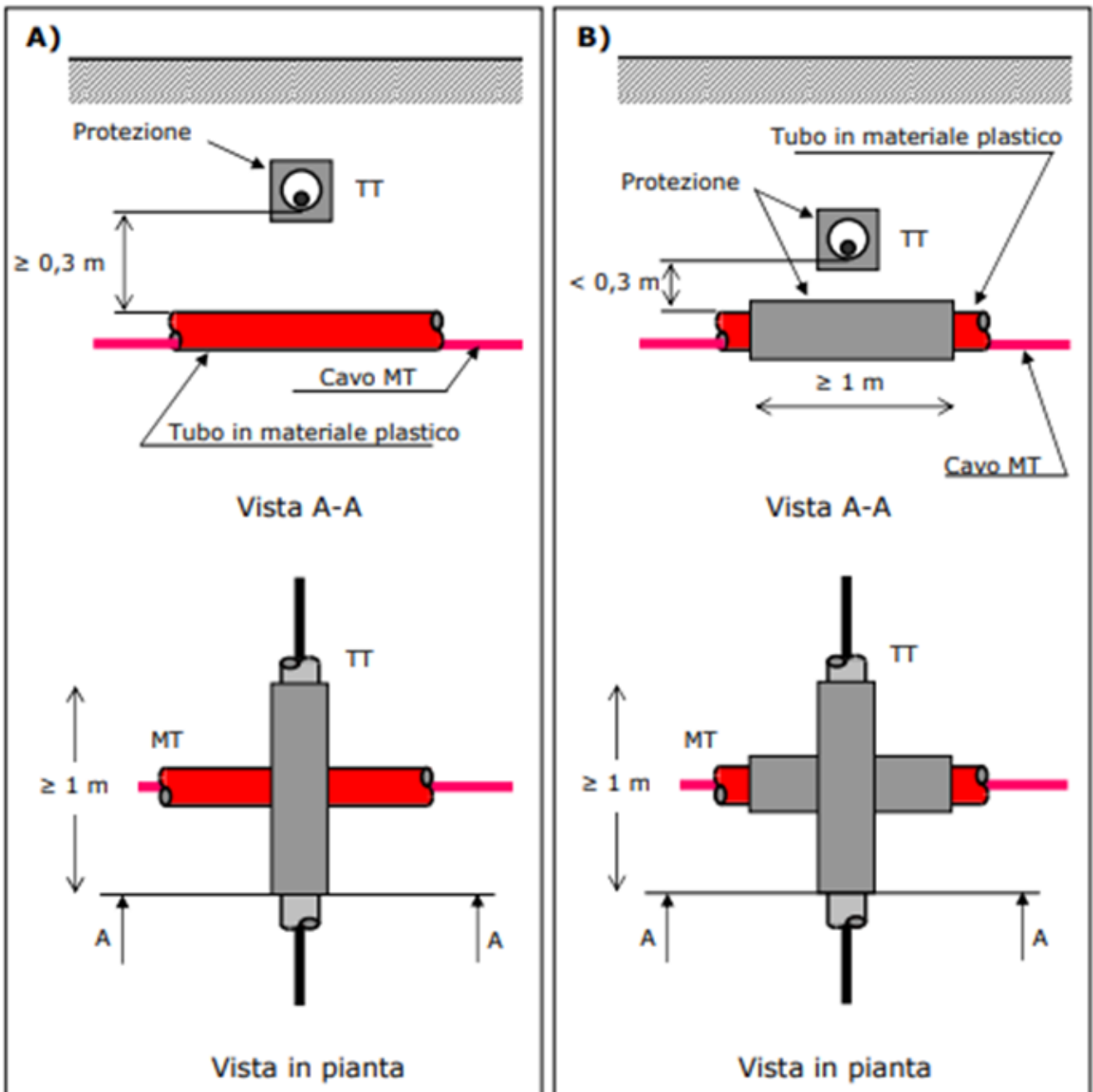
Figura 15- Modalità di risoluzione interferenze con linee di telecomunicazione
