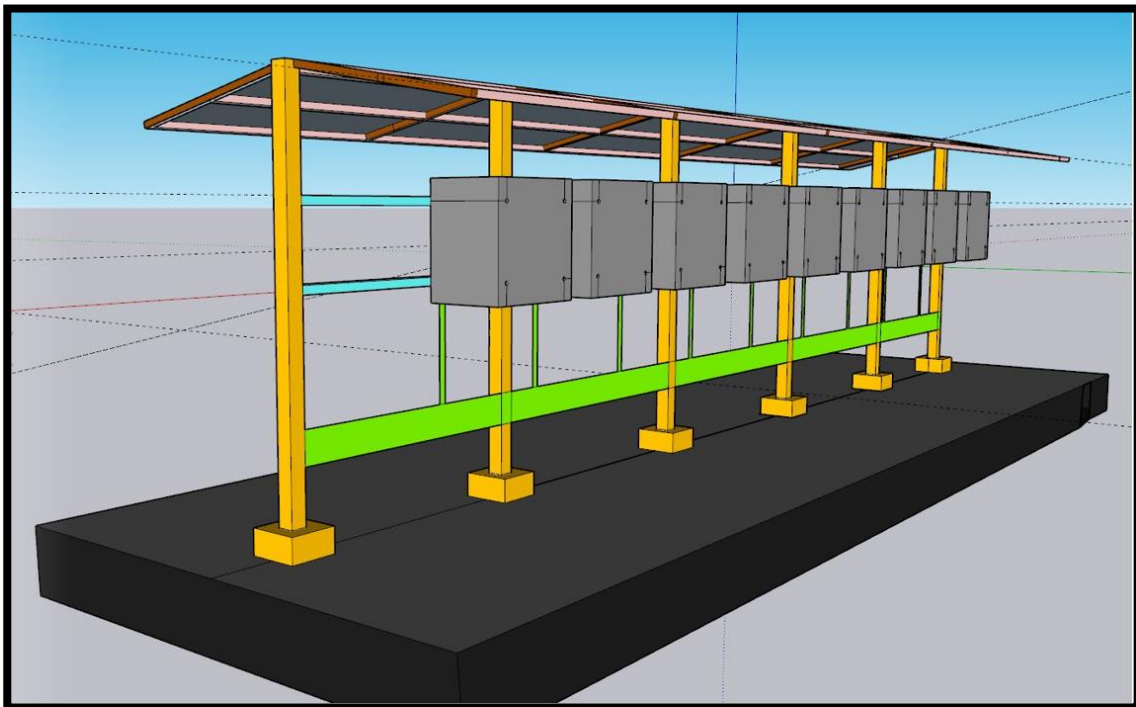
Figure 9 Rastrelliera di ancoraggio inverter
