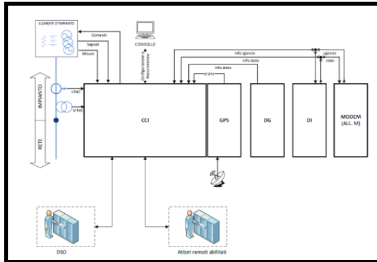
Figura 1 Schema Generale Controllo Centrale di impianto
