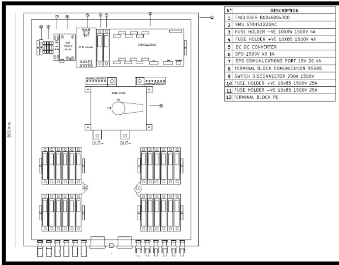
Figure 10 Cassette stringhe intelligenti
