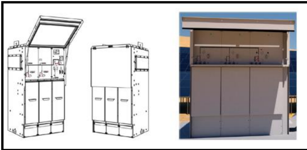
Figure 11 Scoparto MT di sezionamento
