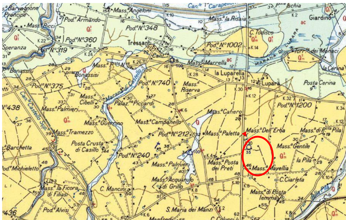
Figura 2: stralcio del foglio 164 della carta geologica con ubicazione dell'area d'intervento
