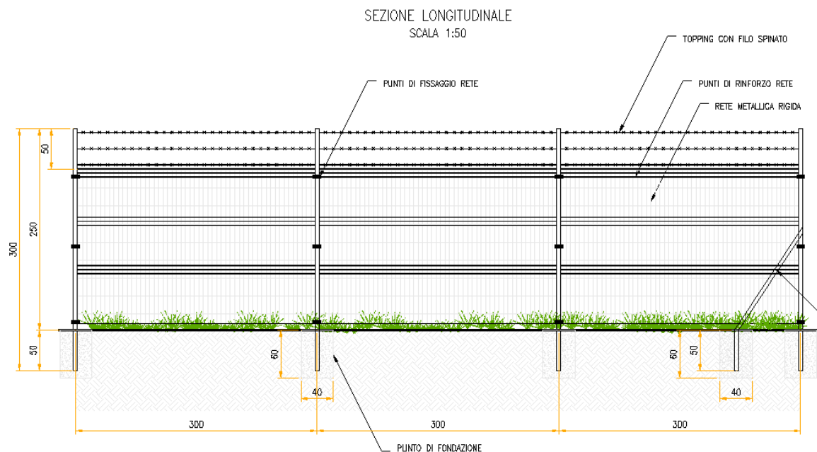
Figura 3.4: Particolare recinzione
