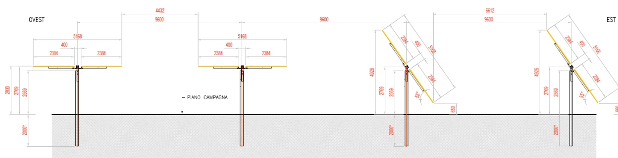
Figura 3.2: Particolare strutture di sostegno moduli
