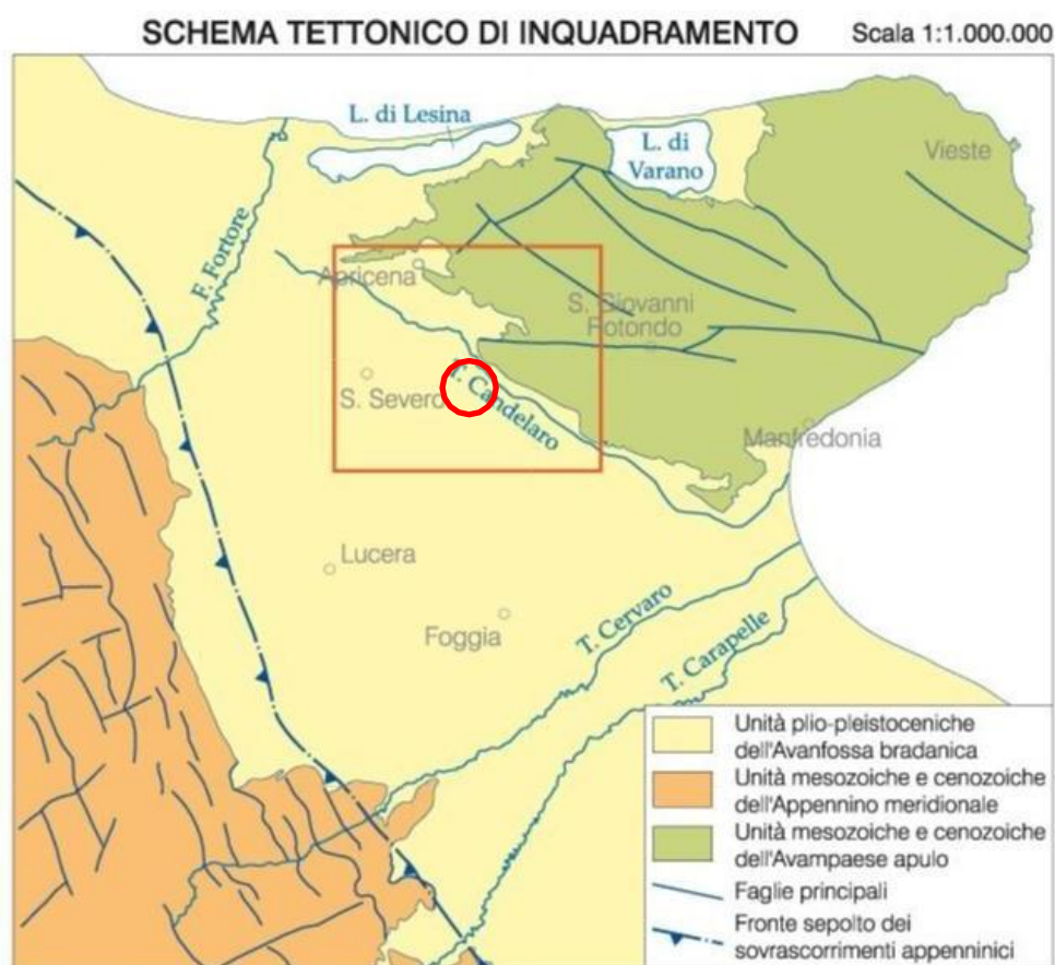
Figura 2.5: Schema geologico e strutturale dell'area del Tavoliere e del Subappennino Dauno – Area di cantiere nel cerchio rosso.
