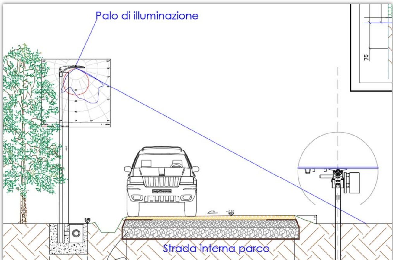
Fig. 8. Schematizzazione della distribuzione del fascio luminoso per la sorgente di progetto, nei tratti in prossimità delle strade di servizio.
