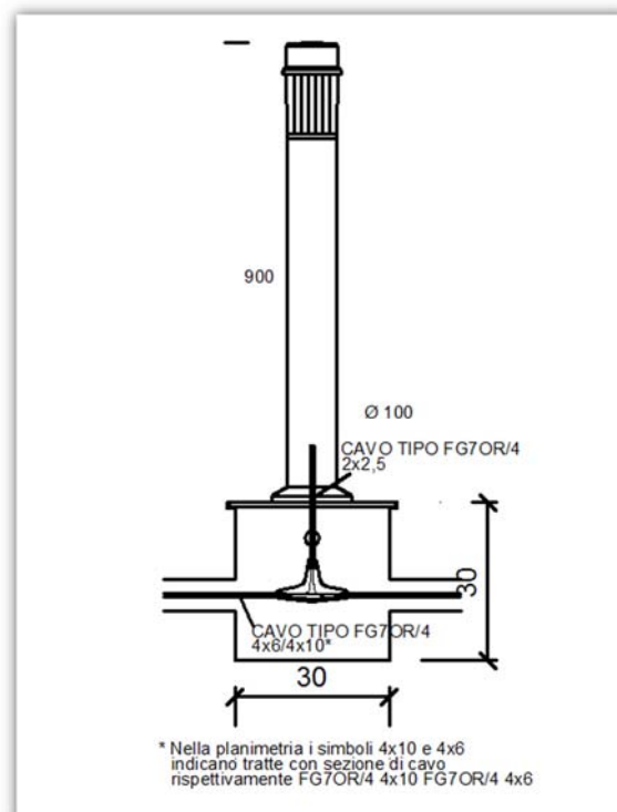
Fig. 6. – Illuminazione per viabilità interna.
