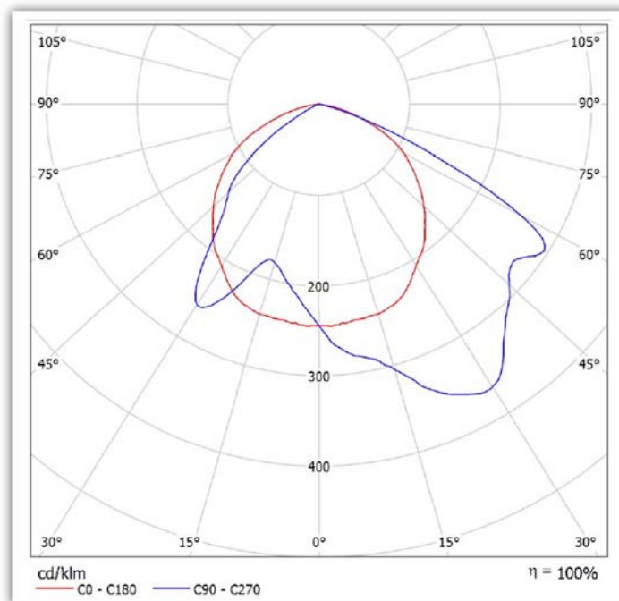
Fig. 4. Fotometrica calcolata per il proiettore di progetto, con corrente di impiego pari a 350mA
