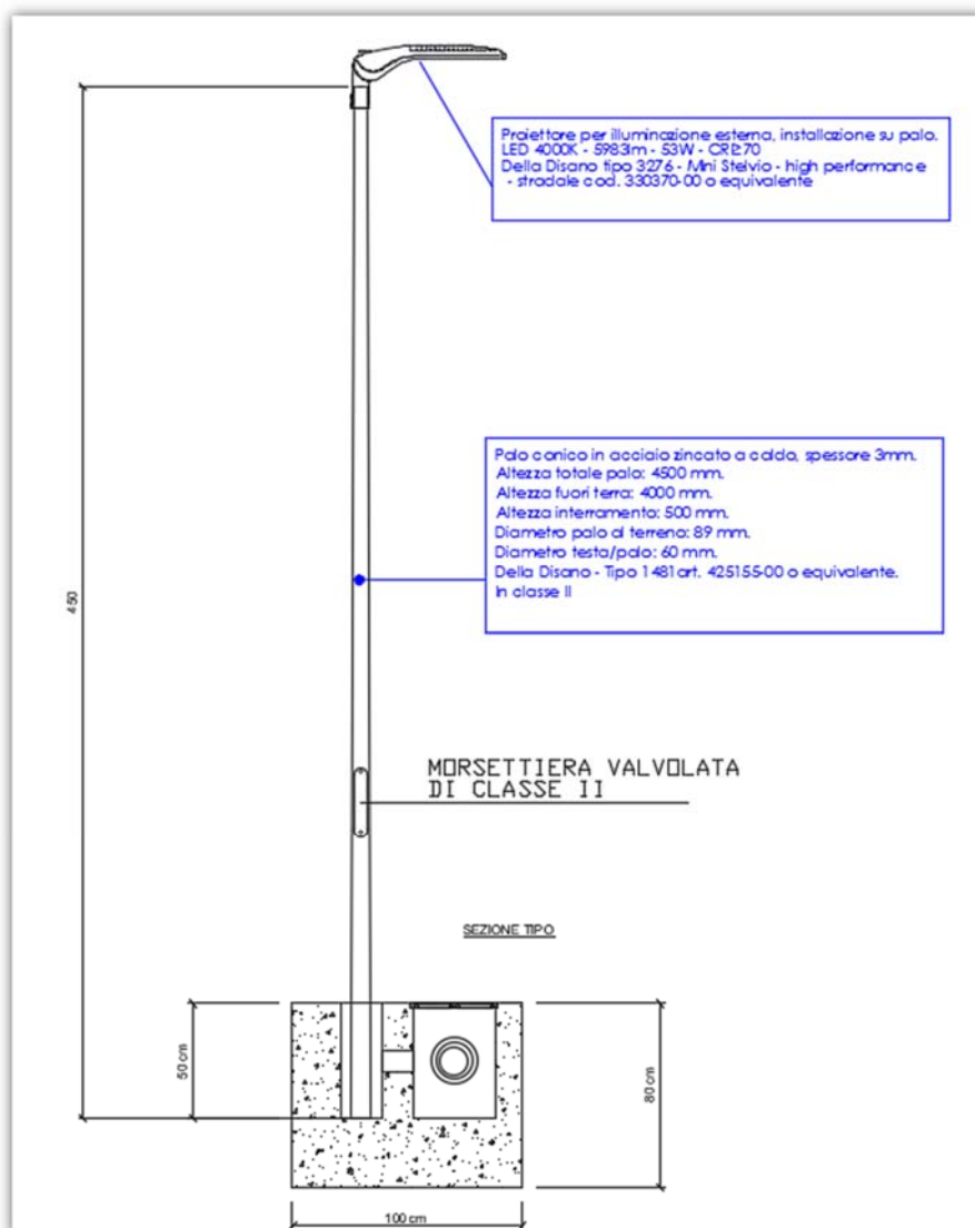
Fig. 2. – Illuminazione perimetrale.
