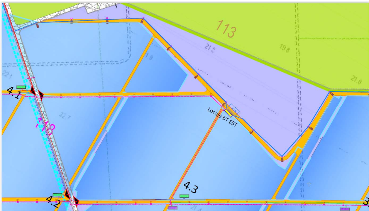
Fig. 1. Dettaglio planimetrico con evidenza della posizione del quadro bT di alimentazione dell'impianto di illuminazione del sottoimpianto EST: lungo la fascia perimetrale in verde sono visibili le armature stradali su palo alto, alimentate mediante linea bT con tratto blu; lungo la viabilità interna sono posizionati i pali segnapasso, rappresentati con cerchio rosso, ed alimentati da linea bT con tratto magenta;
