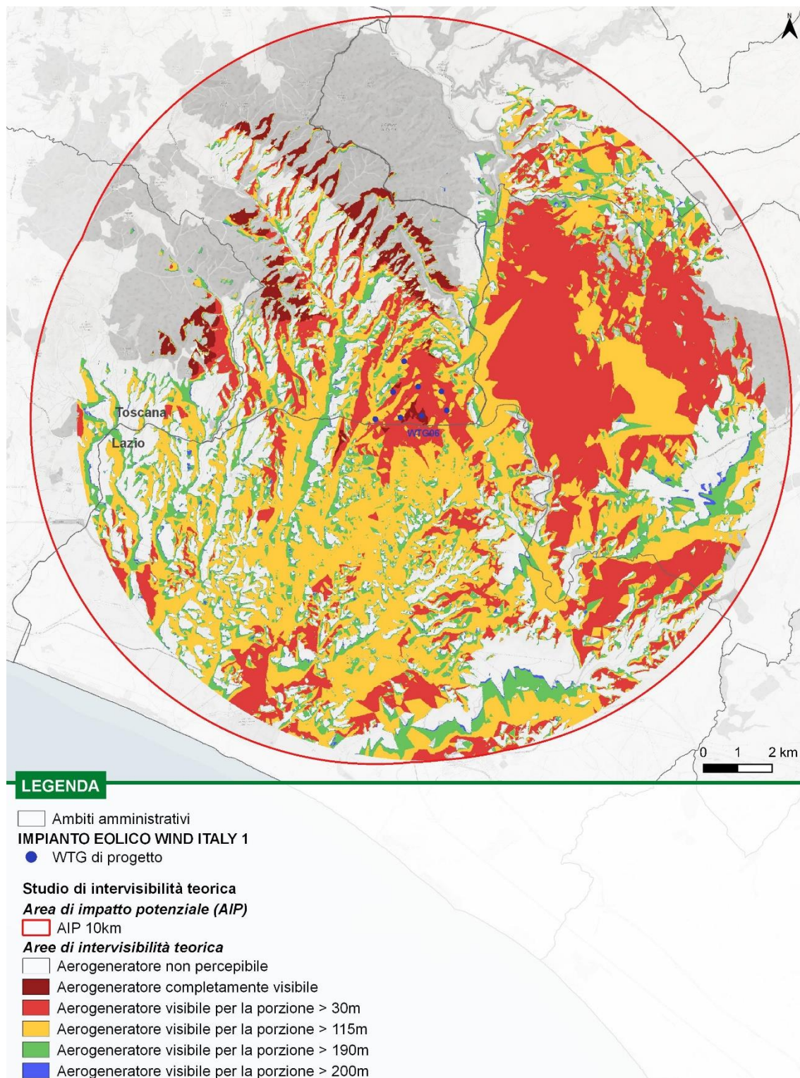
Figura 5.14: Interisibilità dell'aerogeneratore 06
