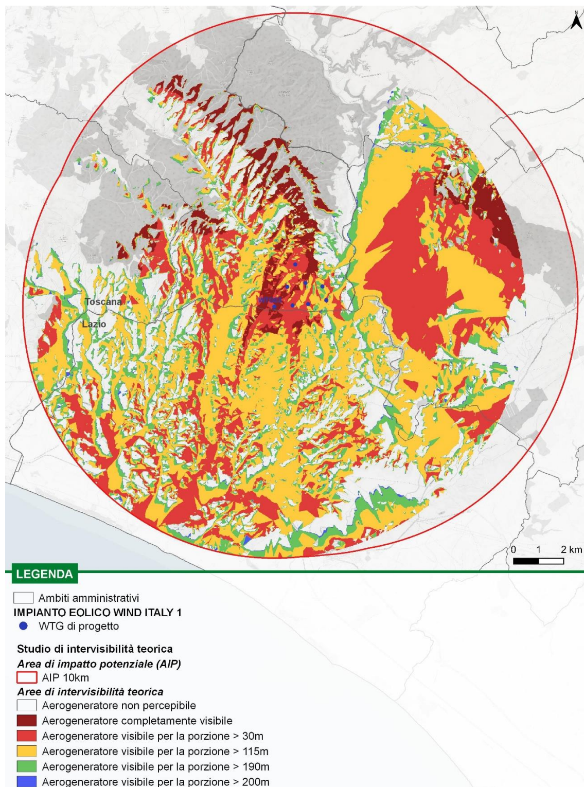
Figura 5.11: Interisibilità dell'aerogeneratore 03
