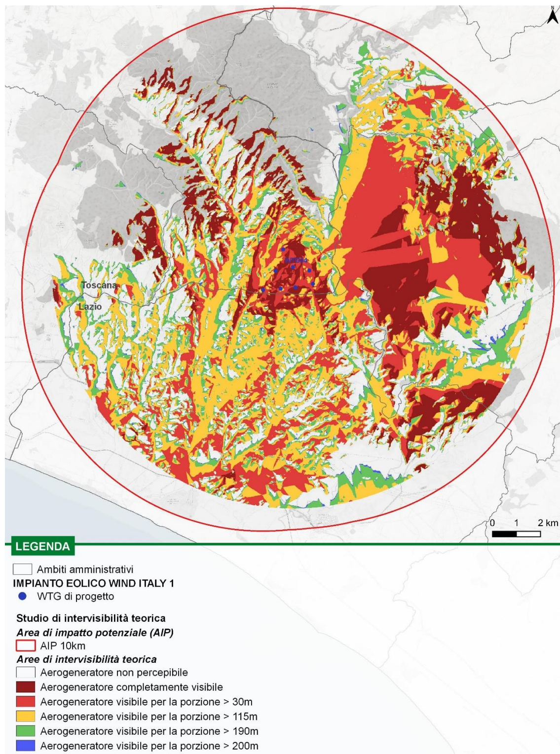
Figura 5.12: Intervisibilità dell'aerogeneratore 04
