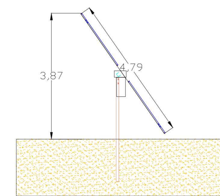
Inseguitore monossiale - Vista laterale con inclinazione a 55°
