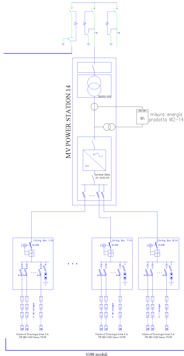
FIGURA 5 - SCHEMA ELETTRICO SOTTOCAMPO
