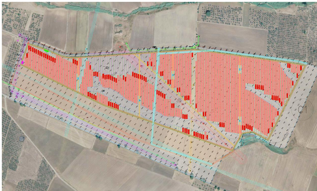
Figura 3.1: Layout di progetto.
