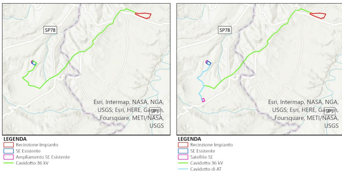
Figura 3.6: Soluzioni di Connessione alla SE 380/150 "Rotello"
