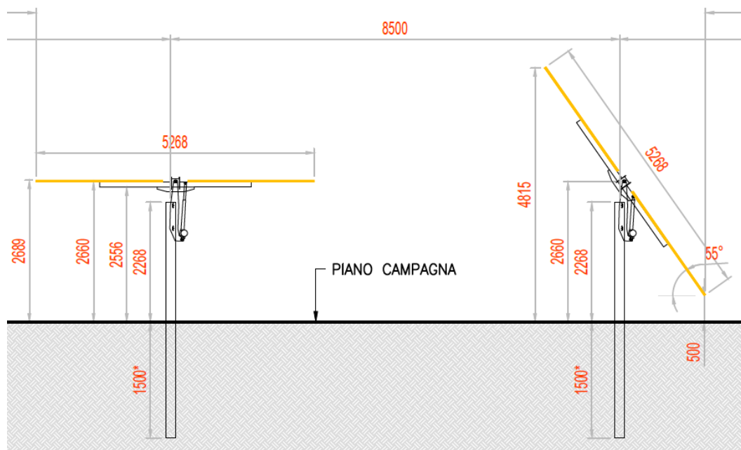
Figura 3.2: Particolare strutture di sostegno moduli
