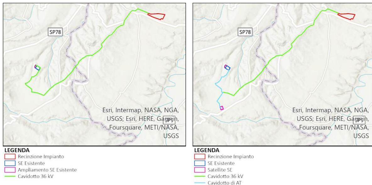
Figura 3.1: Soluzioni di Connessione alla SE 380/150 "Rotello"
