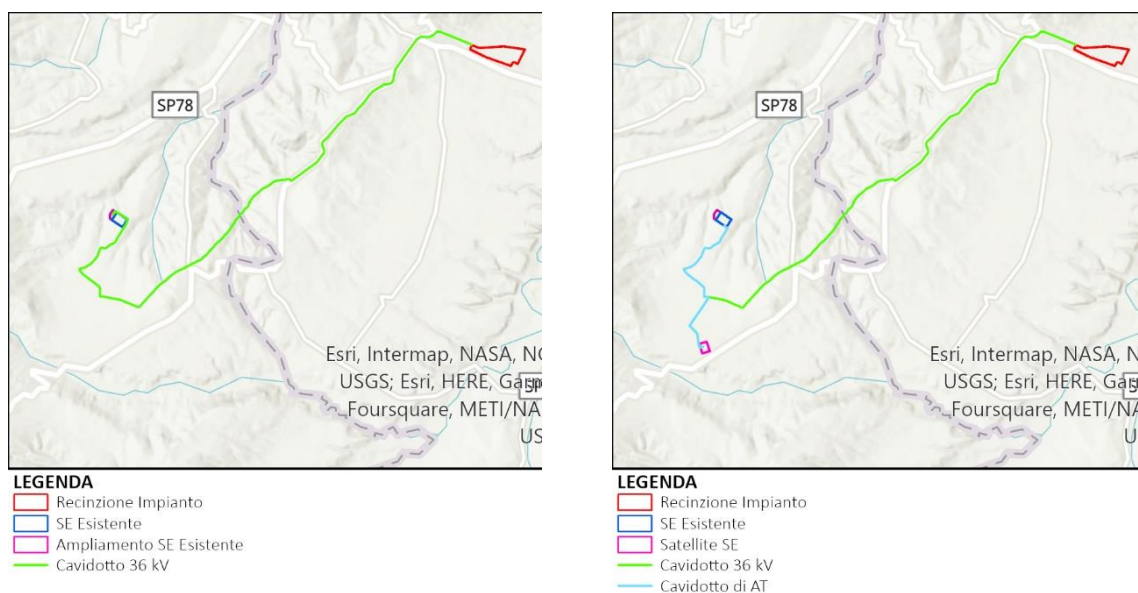
Figura 2.3: Soluzioni di Connessione alla SE 380/150 "Rotello"
