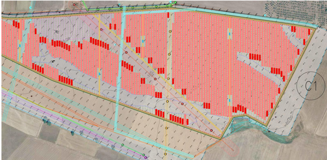
Figura 3.2: Layout con dettaglio interferenze
