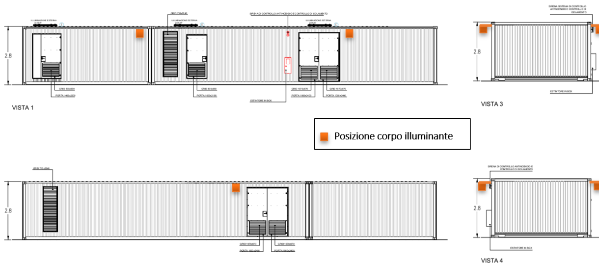
Figura 3.2: Tipologico Cabina di smistamento con indicazione della posizione dei corpi illuminanti
