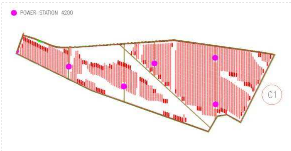
Fig. 2: Layout impianto
