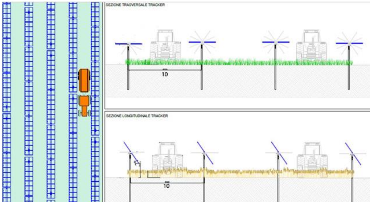
Figura 8 – Planimetrie e sezioni tracker
