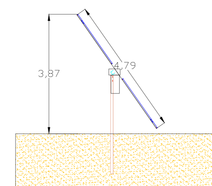
Inseguitore monossiale - Vista laterale con inclinazione a 55°
