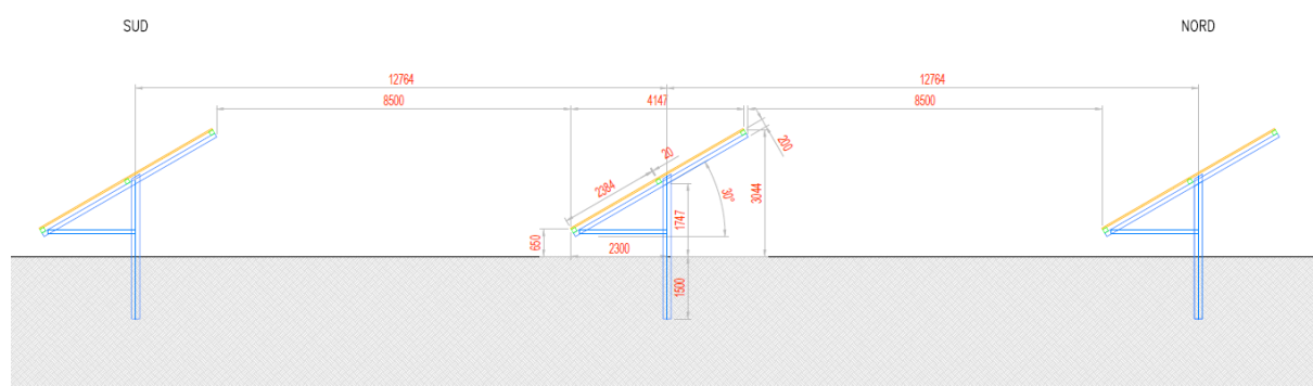
Figura 4.2: Particolare strutture di sostegno moduli fissi
