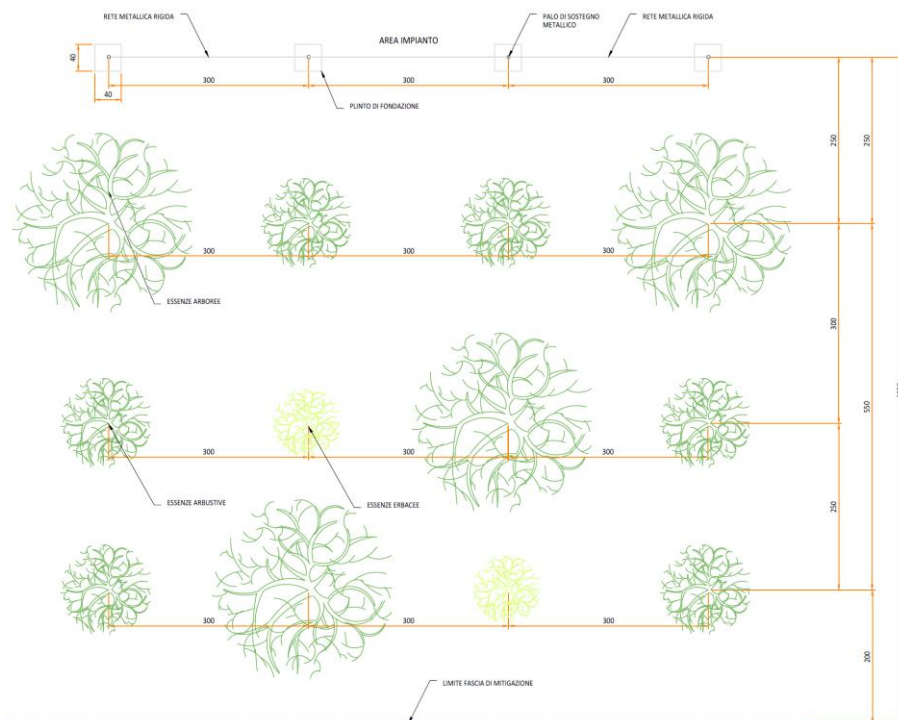
Figura 4.14: Tipologico del Filare di Mitigazione
