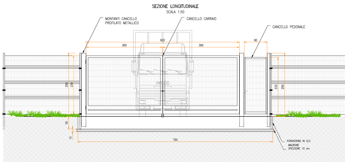
Figura 4.5: Particolare accesso
