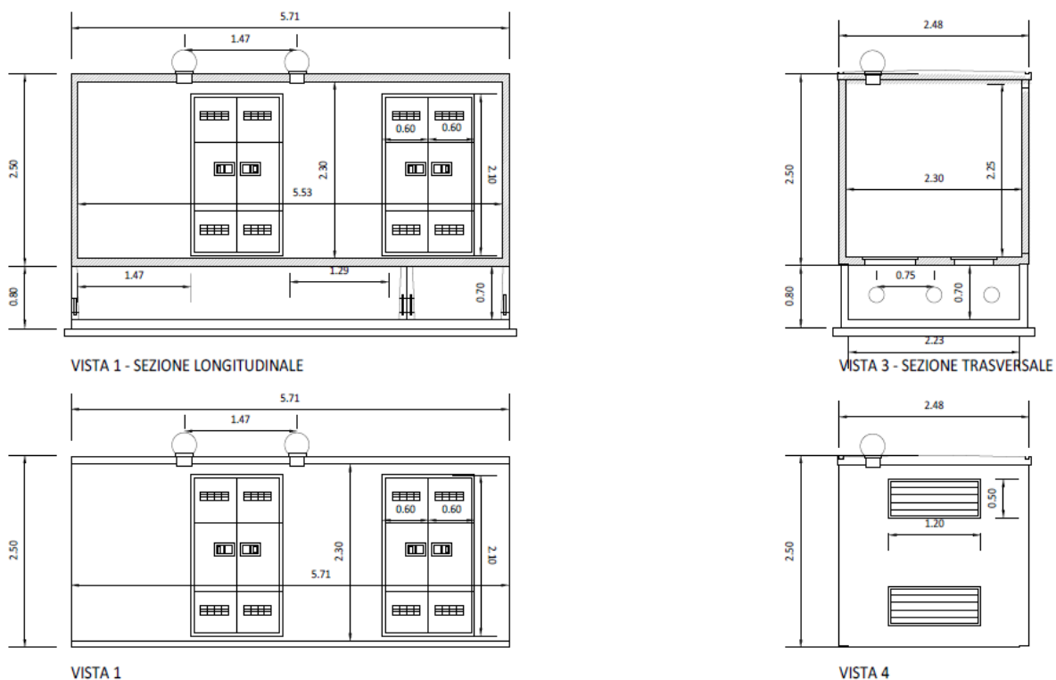
Figura 4.20: Prospetti rappresentativi delle Cabine di Sezionamento
