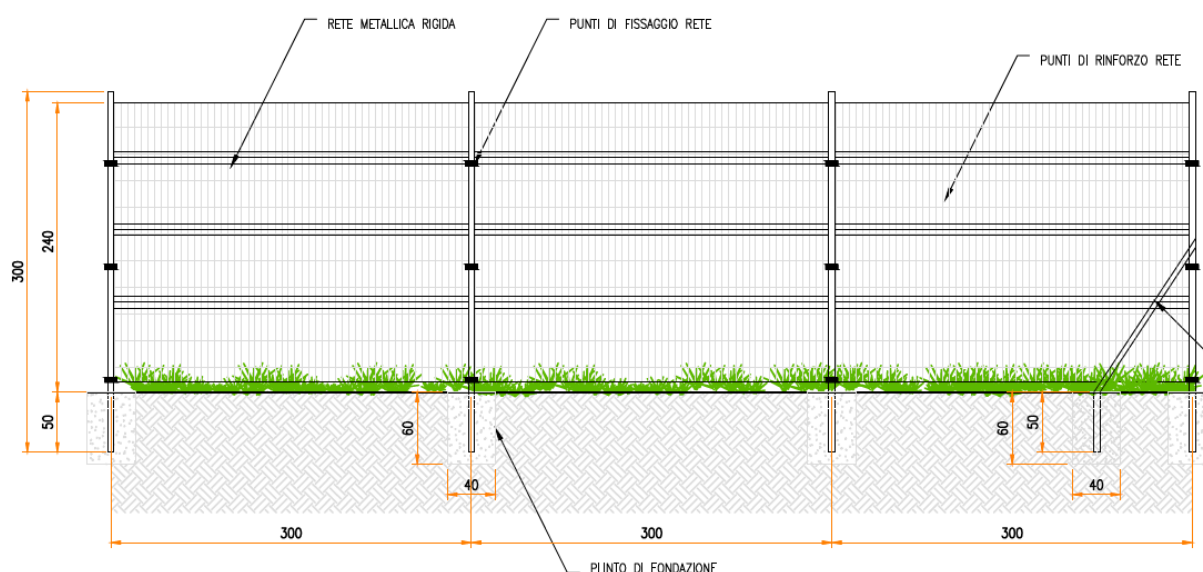
Figura 4.4: Particolare recinzione
