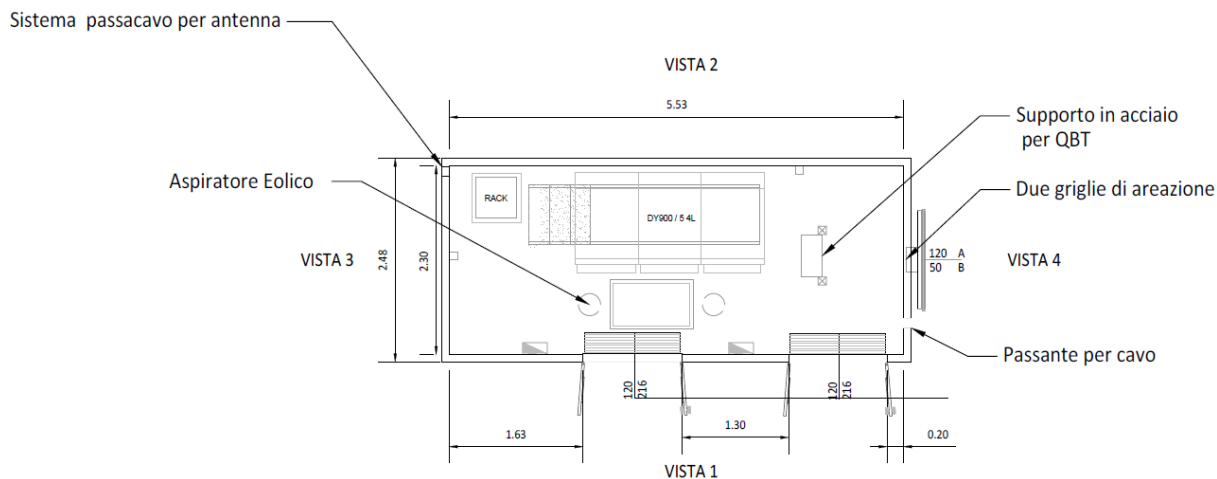
Figura 4.19: Planimetria Cabine di Sezionamento
