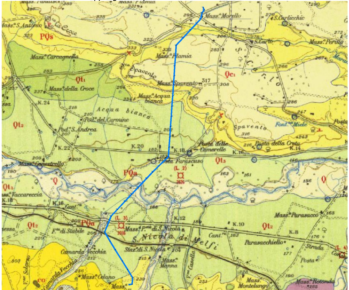
Estratto della carta geologica d'Italia, F. 175.
