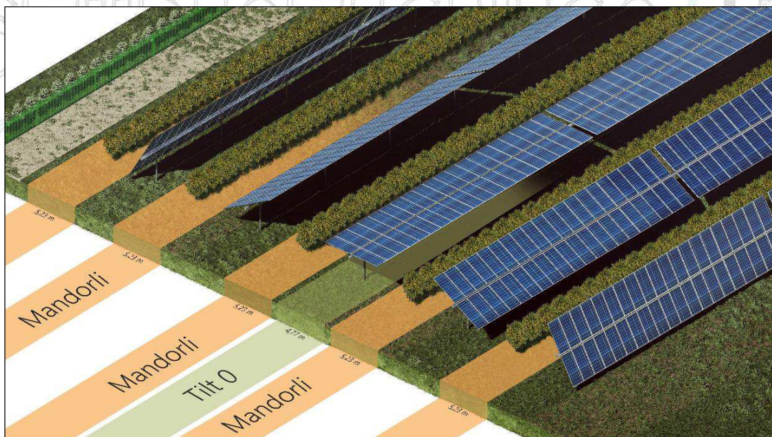
Tav. 30 - Coltivazioni del mandorlo in soluzione agrovoltaico con i moduli alle varie inclinazioni
