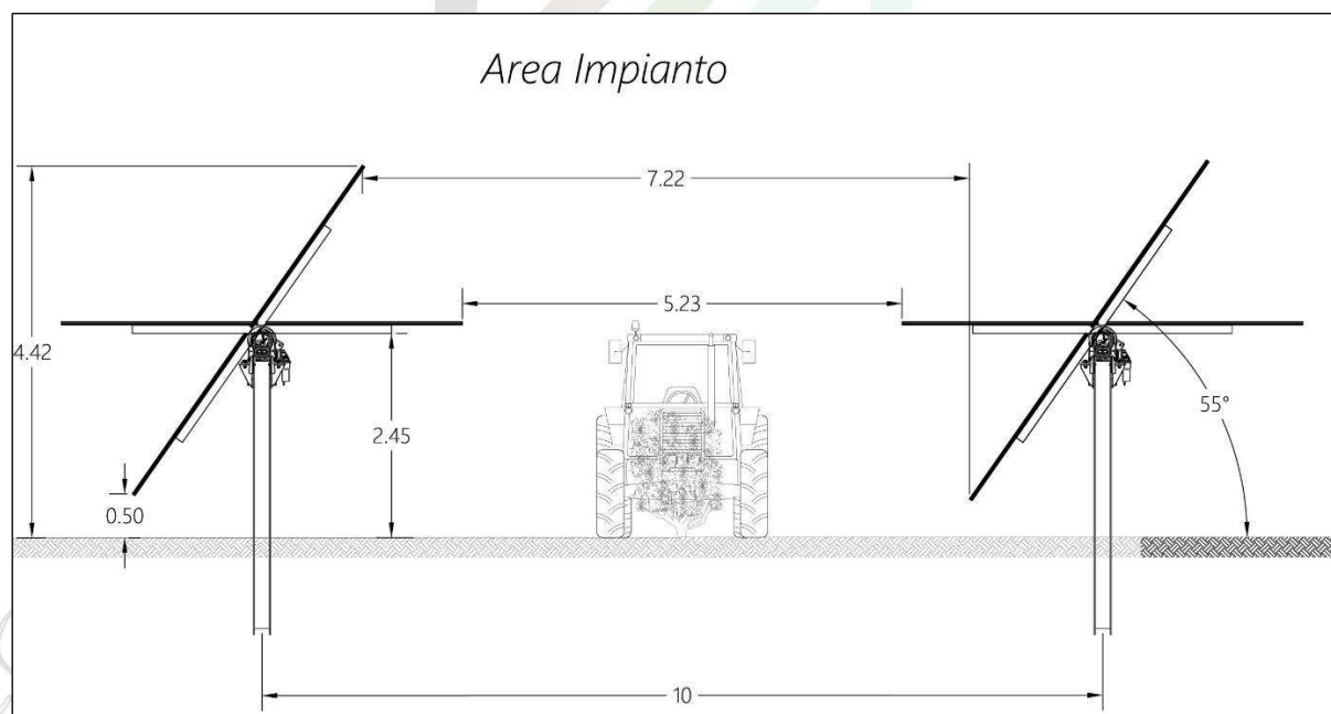
Tav. 18 - Prospetto trasversale (visuale est-ovest)
