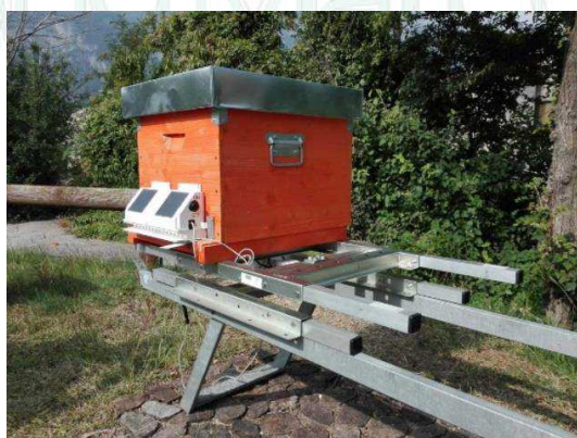
Fig.15 - Esempio di sistema monitoraggio Melixa
