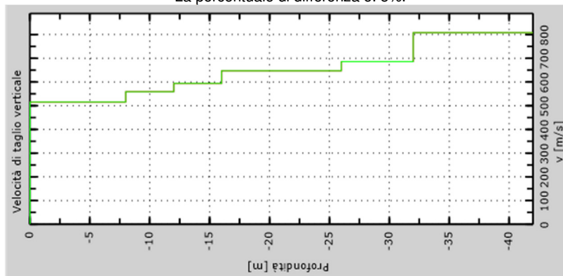
Fig.26 - Profilo verticale delle velocità delle Onde registrate
