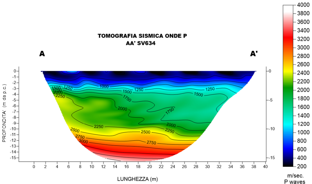
Fig. 9 – Sezione tomografica del profilo AA'
