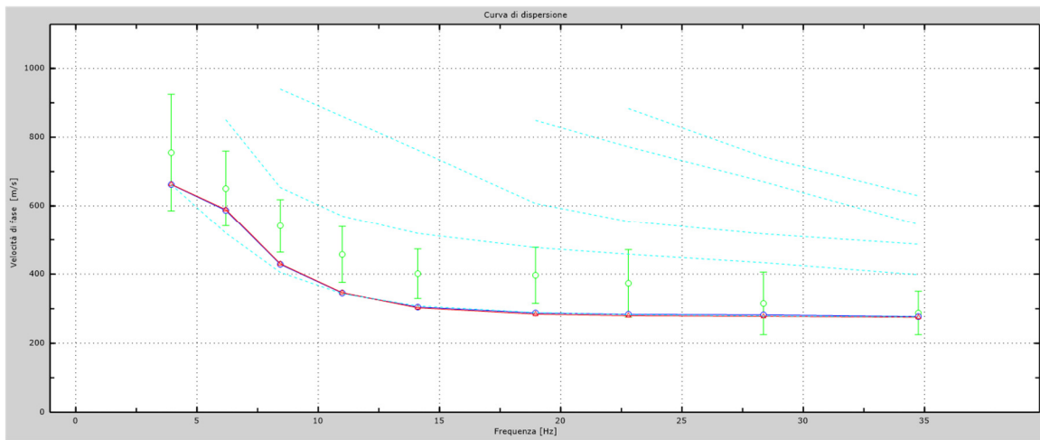
Fig.36 - Curva di dispersione sperimentale.
