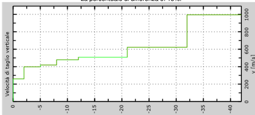
Fig.42 - Profilo verticale delle velocità delle Onde registrate
