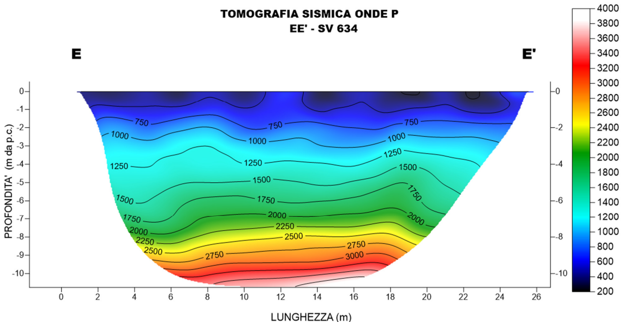
Fig. 21 – Sezione tomografica del profilo EE'
