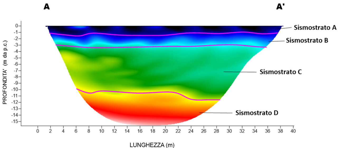
Fig. 10 – Interpretazione sezione tomografica del profilo AA'
