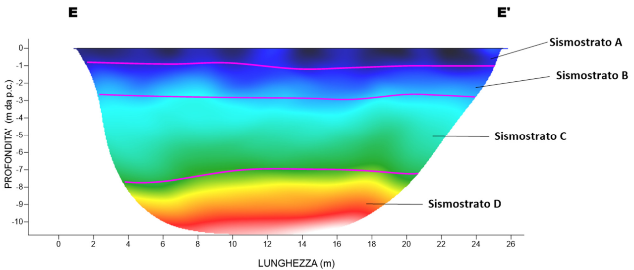
Fig. 22 – Interpretazione sezione tomografica del profilo EE'
