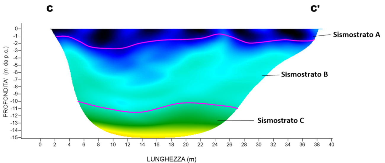
Fig. 16 – Interpretazione sezione tomografica del profilo CC'
