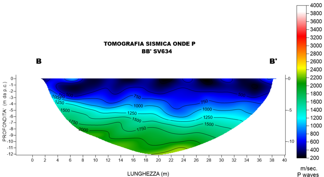
Fig. 12 – Sezione tomografica del profilo BB'
