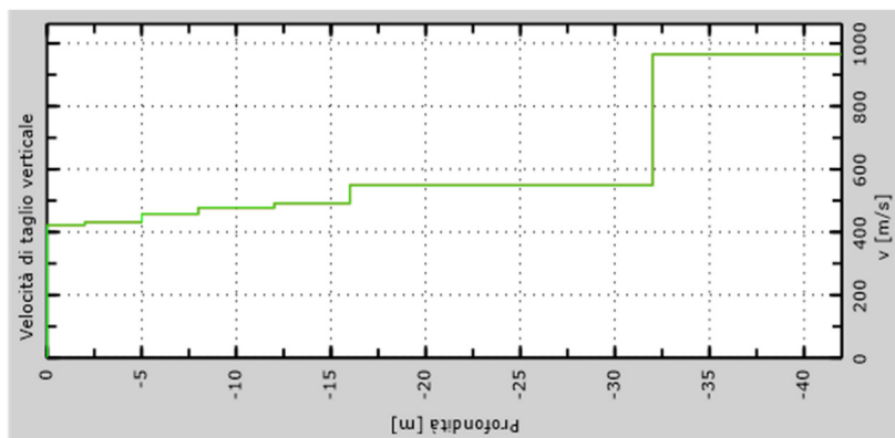
Fig.34 – Profilo verticale delle velocità delle Onde registrate
