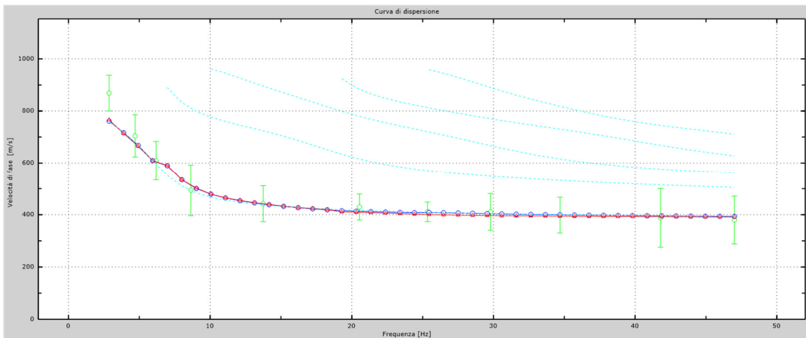
Fig.33 - Velocità numeriche – punti sperimentali (verde), modi di Rayleigh (ciano), curva apparente (blu), curva numerica (rosso). La percentuale di differenza è: 7%.
