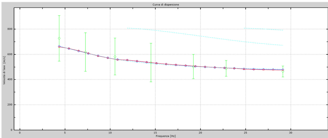
Fig.25 - Velocità numeriche – punti sperimentali (verde), modi di Rayleigh (ciano), curva apparente (blu), curva numerica (rosso). La percentuale di differenza è: 5%.
