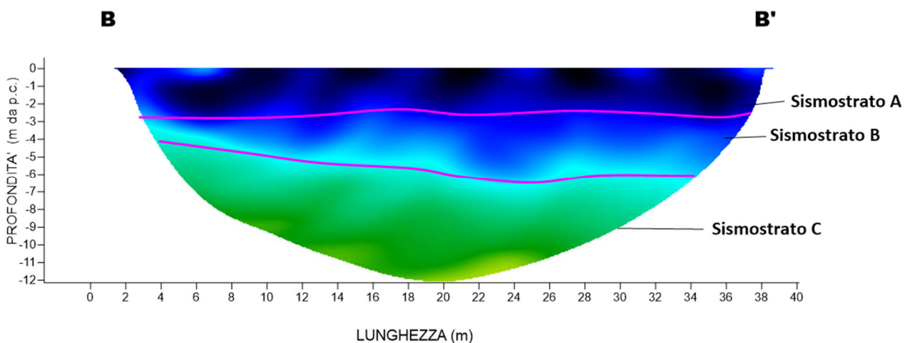
Fig. 13 – Interpretazione sezione tomografica del profilo BB'
