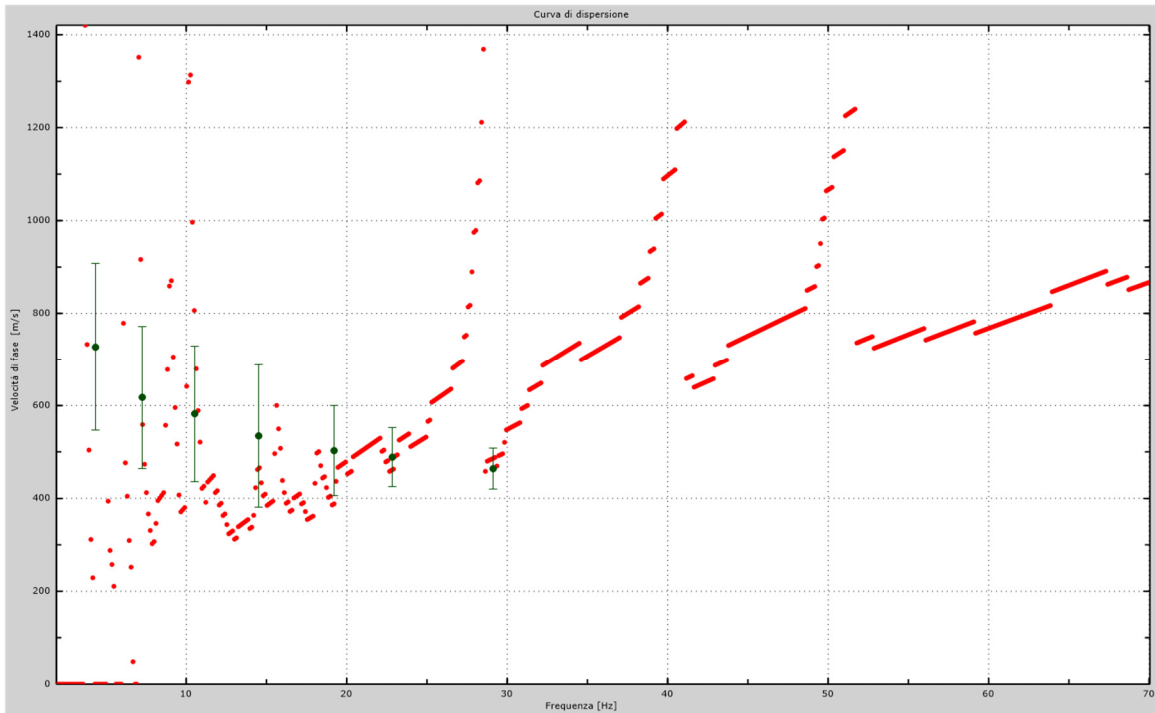
Fig.24 - Curva di dispersione sperimentale.
