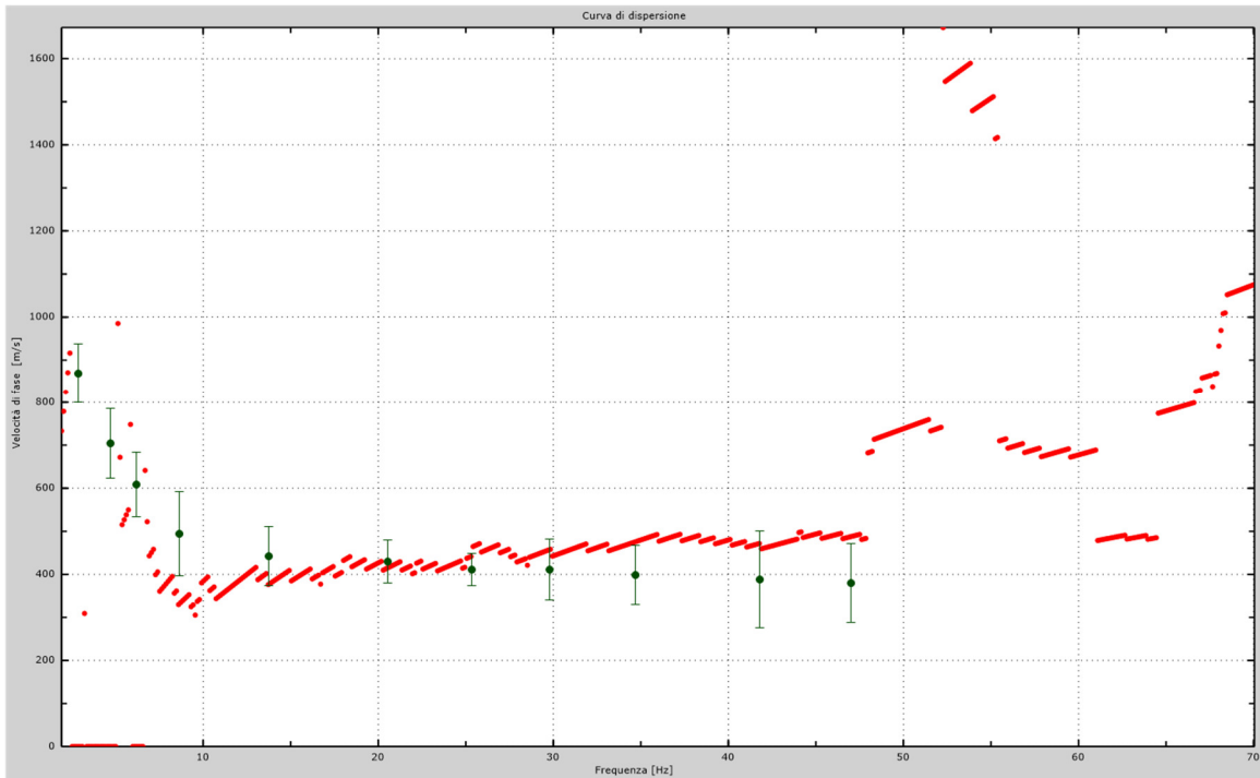
Fig.32 - Curva di dispersione sperimentale.
