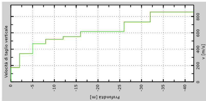
Fig.30 - Profilo verticale delle velocità delle Onde registrate
