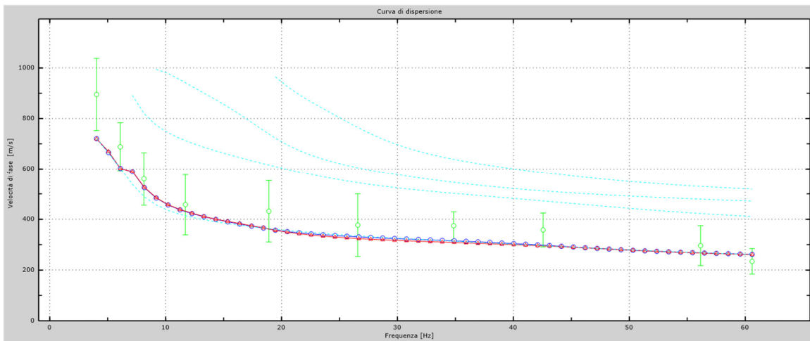
Fig.41 - Velocità numeriche – punti sperimentali (verde), modi di Rayleigh (ciano), curva apparente (blu), curva numerica (rosso). La percentuale di differenza è: 15%.
