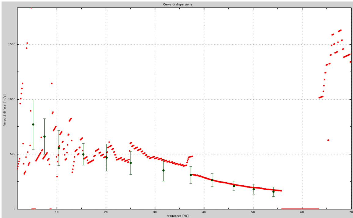
Fig.28 - Curva di dispersione sperimentale.
