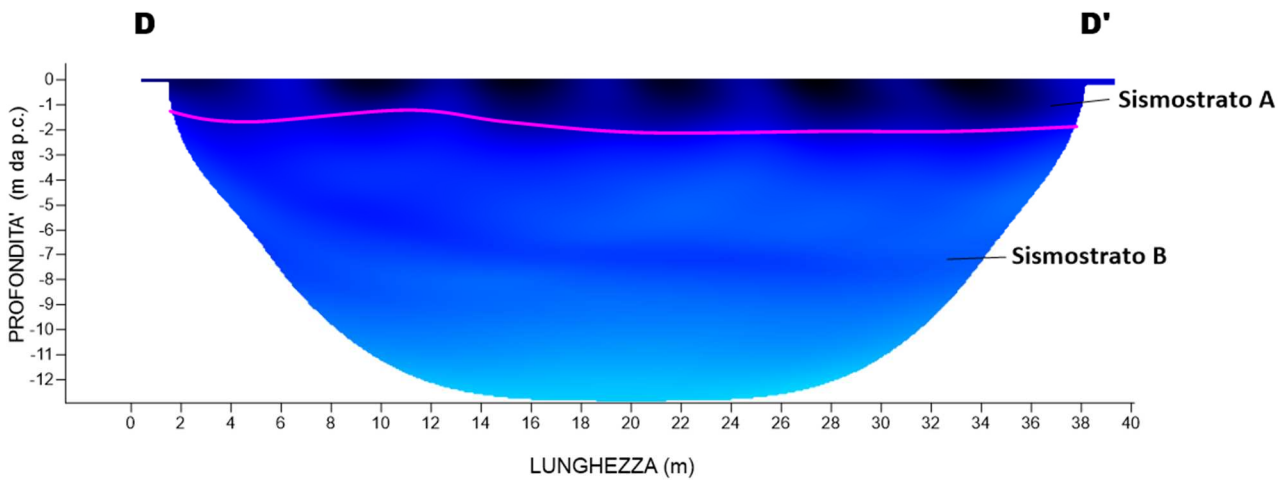
Fig. 19 – Interpretazione sezione tomografica del profilo DD'
