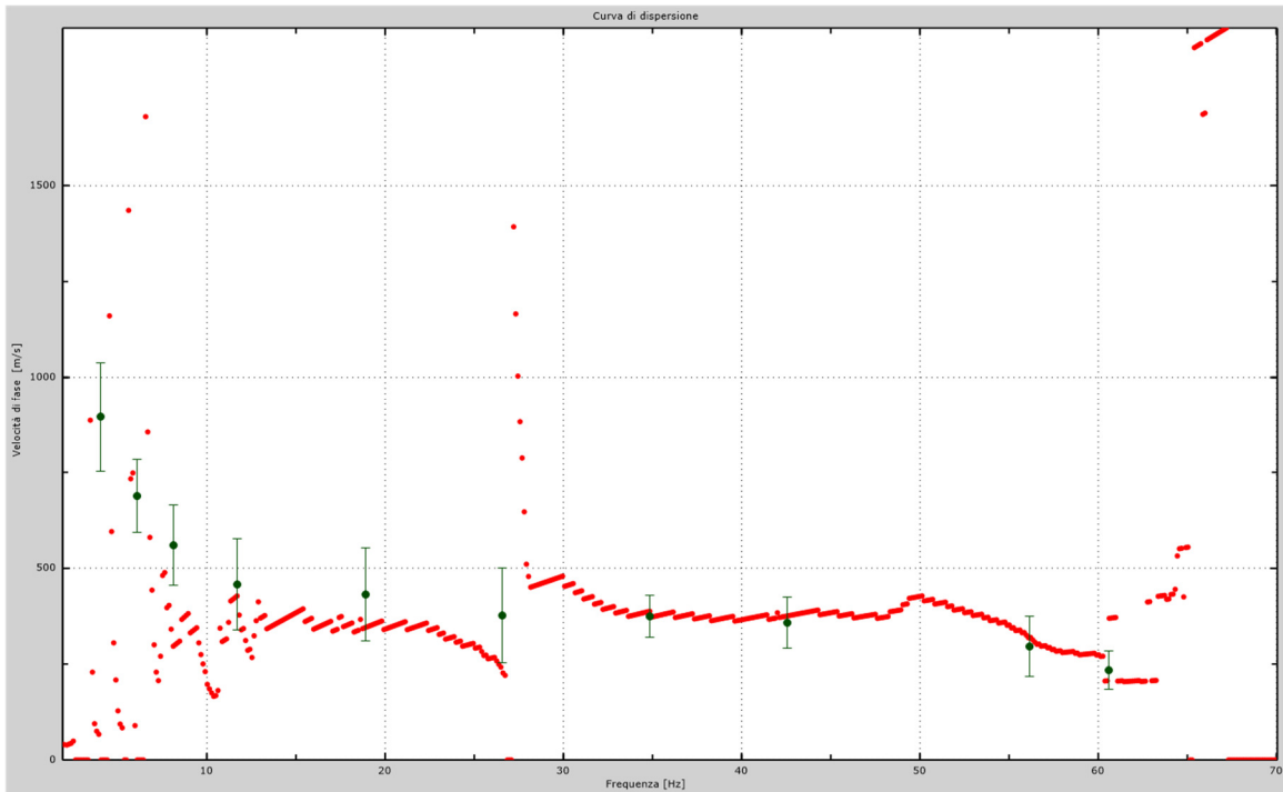
Fig.40 - Curva di dispersione sperimentale.
