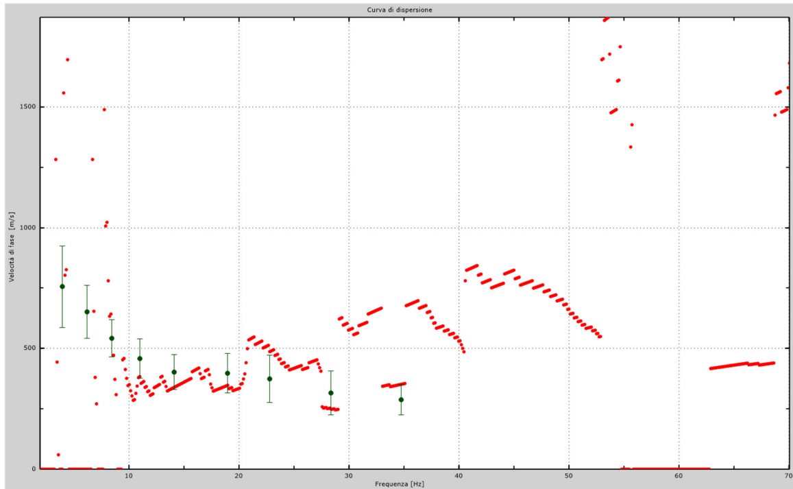
Fig.36 - Curva di dispersione sperimentale.
