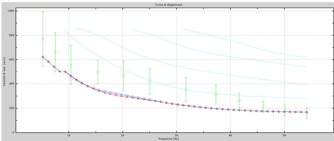
Fig.29 - Velocità numeriche – punti sperimentali (verde), modi di Rayleigh (ciano), curva apparente (blu), curva numerica (rosso). La percentuale di differenza è: 22%.
