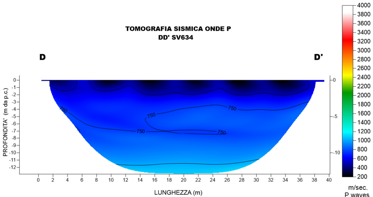
Fig. 18 – Sezione tomografica del profilo DD'
