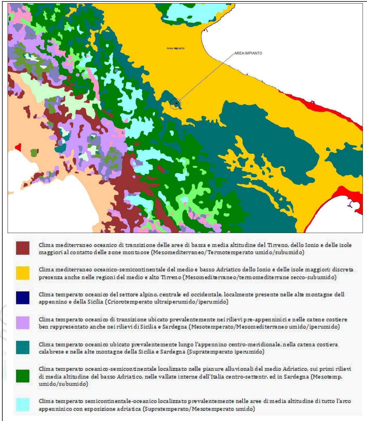
Tav. 11 - Carta Fitoclimatica scala 1: 800.000 (Fonte dati pcn.minambiente.it)
