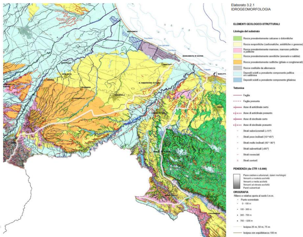
Fig. 2-6: Idrogeomorfologia
