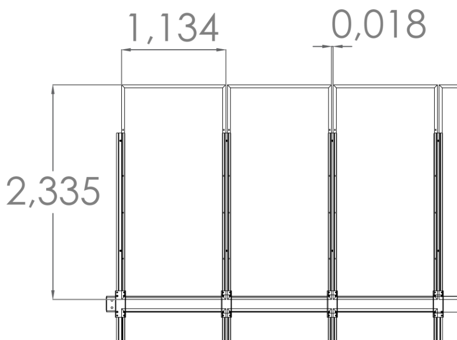
Figura 3-1: Dettaglio Modulo/Tracker
