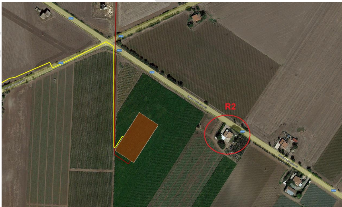
Figura 3-3: Ricettori
