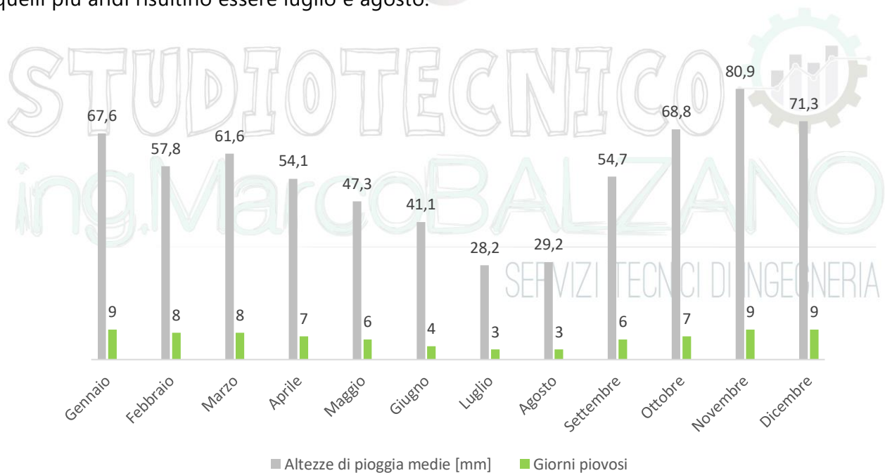
Apporto pluviometrico mensile - stazione di Altamura (1921-2019)
