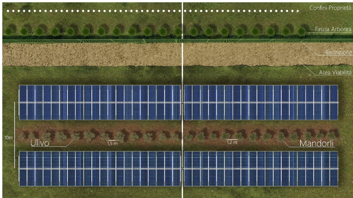
Figura 3-8: Progetto agrivoltaico in progetto
