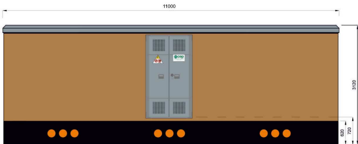
Figura 5 - Cabina elettrica monoblocco prefabbricata - Cabina elettrica generale di impianto
