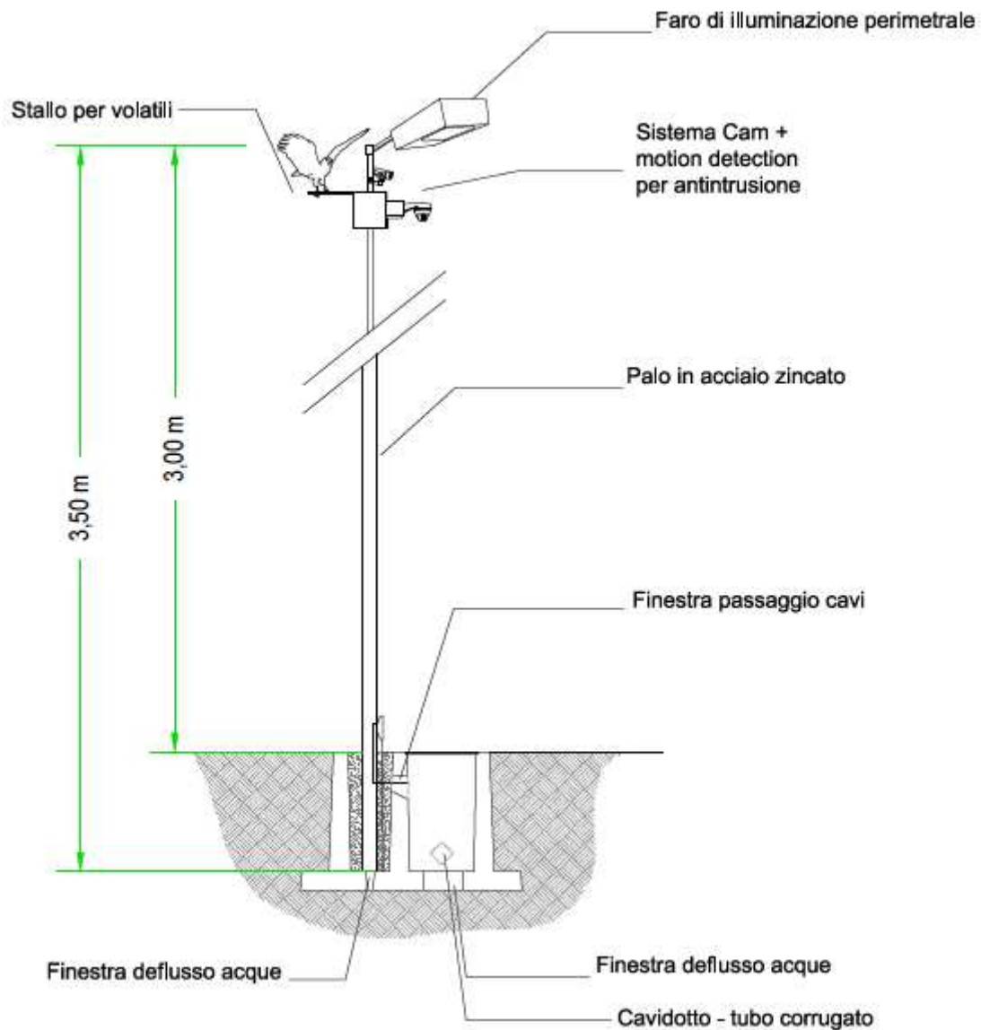
Figura 9 - particolare pali perimetrali di impianto
