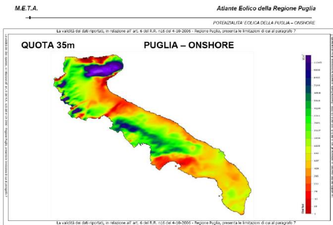
Figure 4-6. Potenzialità eolica della regione Puglia a quota 35 m
