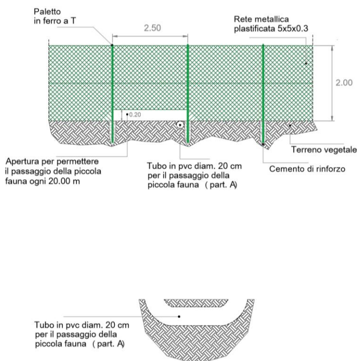
Figure 10-1. Particolare del passaggio della fauna lungo la recinzione perimetrale l'impianto.
