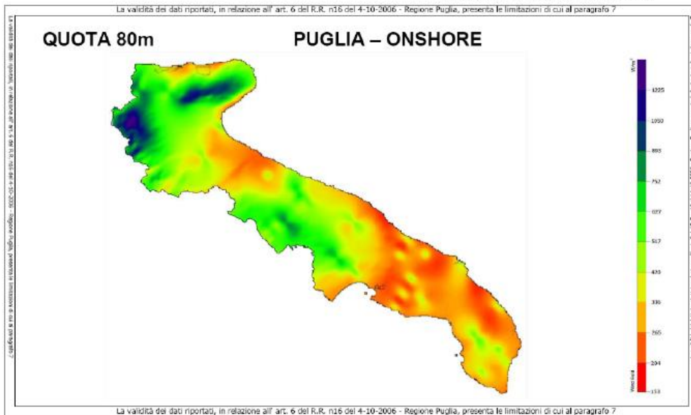
Figure 4-8. Potenzialità eolica della regione Puglia a quota 80 m
