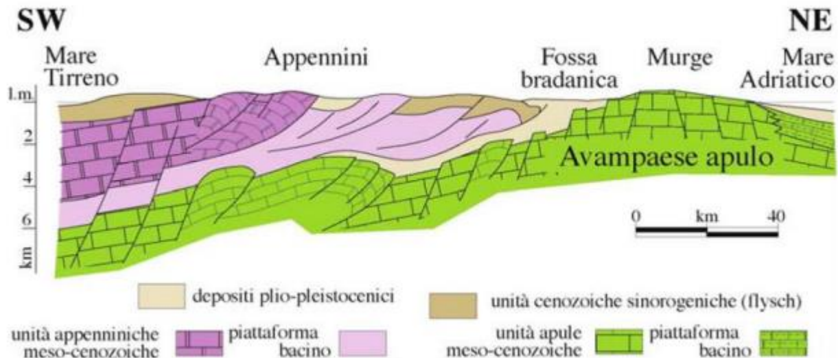
Figure 4-10. sezione trasversale illustrante l'assetto dei domini geostrutturali nel sistema orogenetico appenninico (Tropeano M., 2003)
