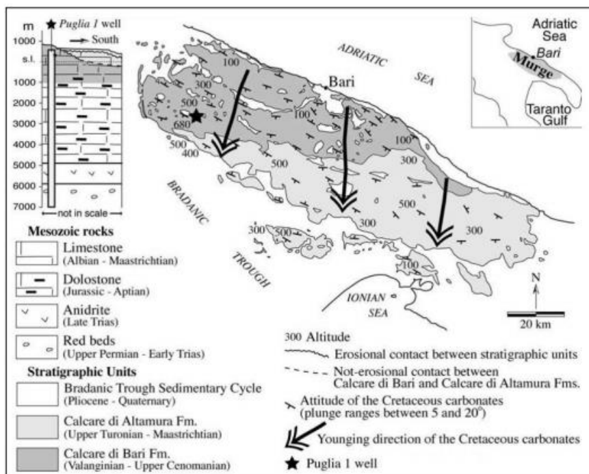
Figure 4-12. Principali unità stratigrafiche nelle Murge e loro relazioni con quelle perforate nel sottosuolo (Festa, 2003)
