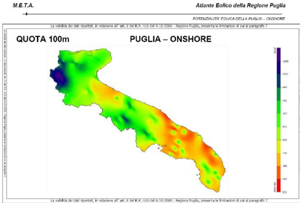
Figure 4-9. Potenzialità eolica della regione Puglia a quota 100 m
