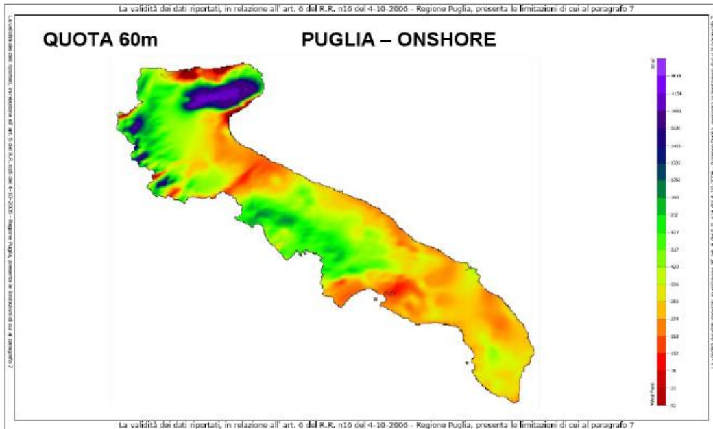
Figure 4-7. Potenzialità eolica della regione Puglia a quota 60 m
