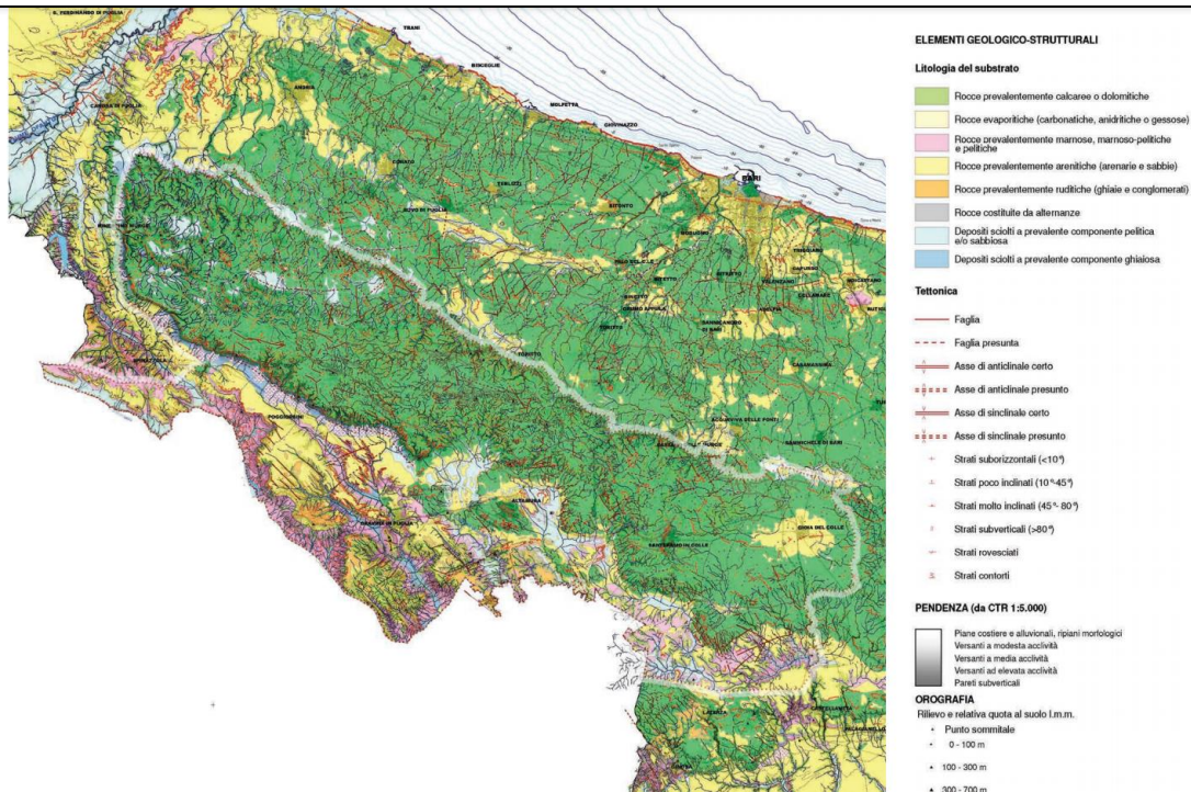
Figure 4-11. elementi geologico-strutturali da sitografia -
