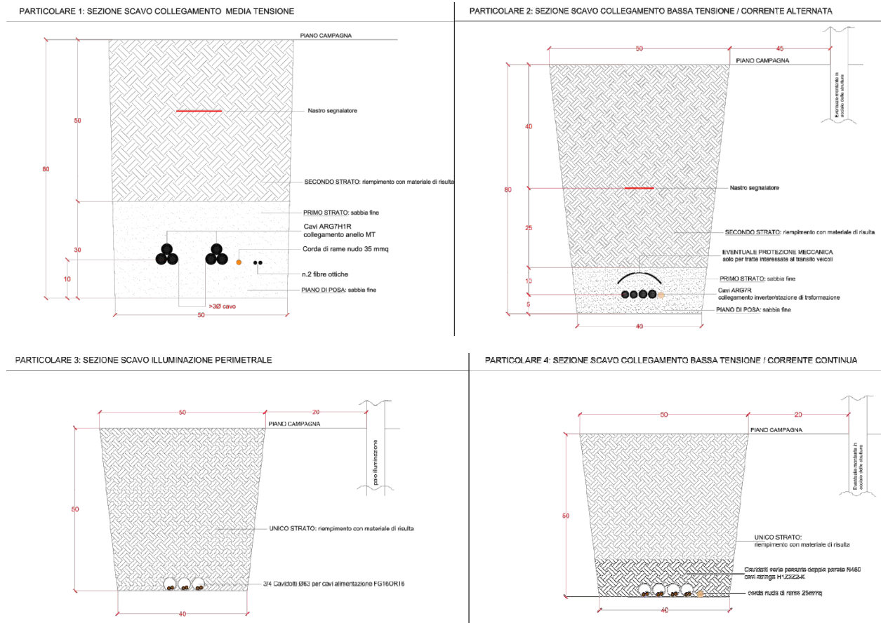
Figura 4-3: particolare dei cavi interni alle aree del parco fotovoltaico
