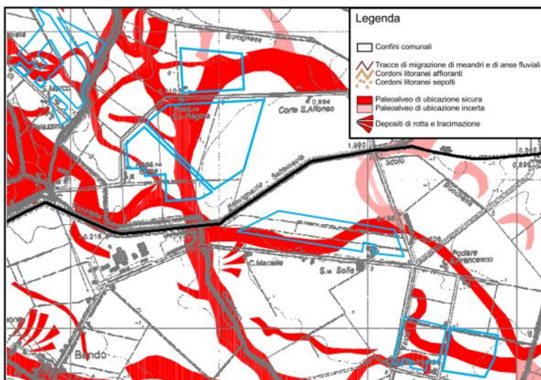
Figura 3-7: Inquadramento geomorfologico del territorio comunale di Argenta, con ubicazione dell'area in esame (rettangolo azzurro), tratto dalla carta geomorfologica a supporto del PSC.
