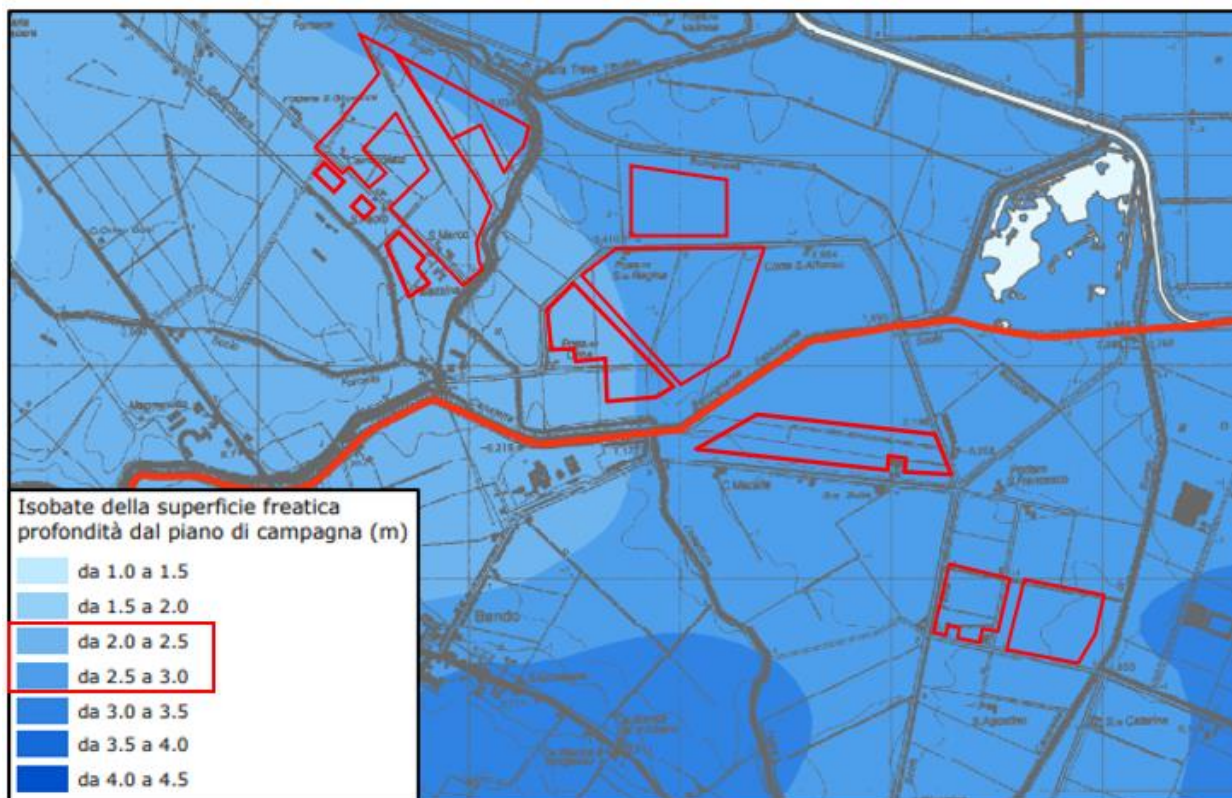
Figura 3-9 Estratto dalla Carta delle Isobate, a supporto del PSC di “Unione dei Comuni Valli e Delizie”, con ubicazione delle aree in oggetto (rettangoli rossi).
