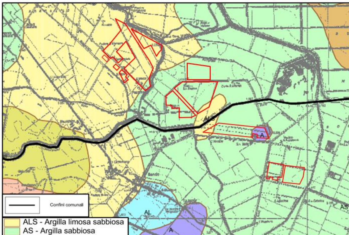
Figura 3-4: Inquadramento geologico del territorio comunale di Argenta, con ubicazione dell'area in esame (rettangolo rosso), tratto dallo studio geologico a supporto del PSC.
