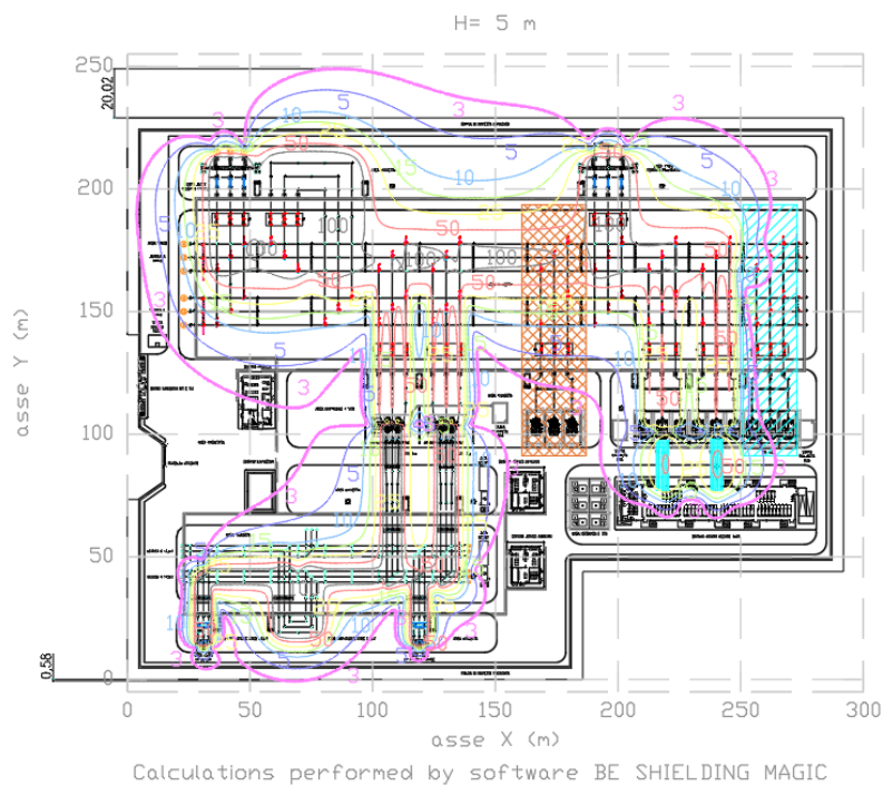
Figura 8 – Livelli di campo magnetico a 5 m dal piano della stazione
