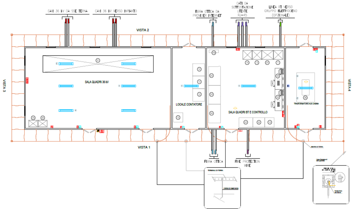
FIGURA 20: ALLESTIMENTO TIPO CABINA DI RACCOLTA
