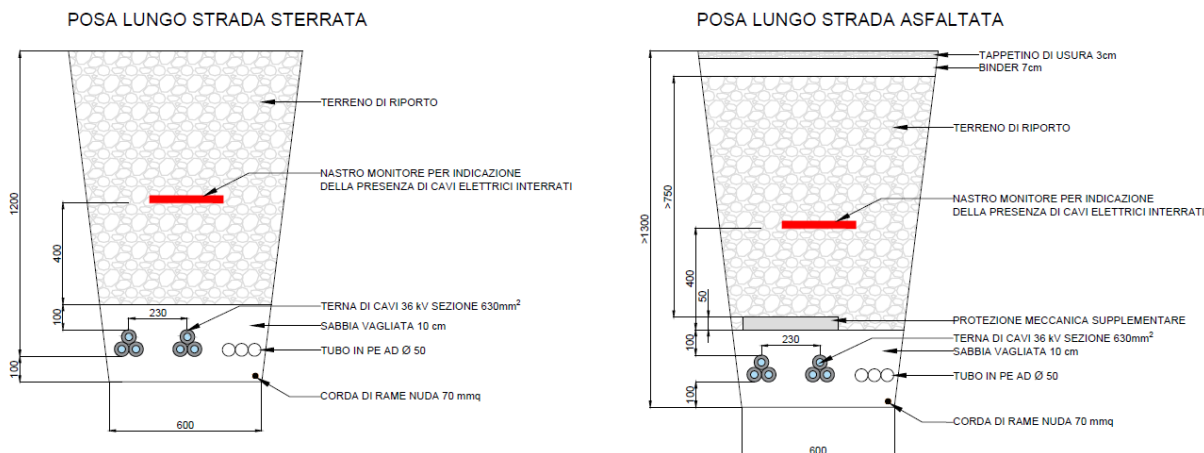
FIGURA 18: TIPOLOGICO POSA LINEE DI CONNESSIONE
