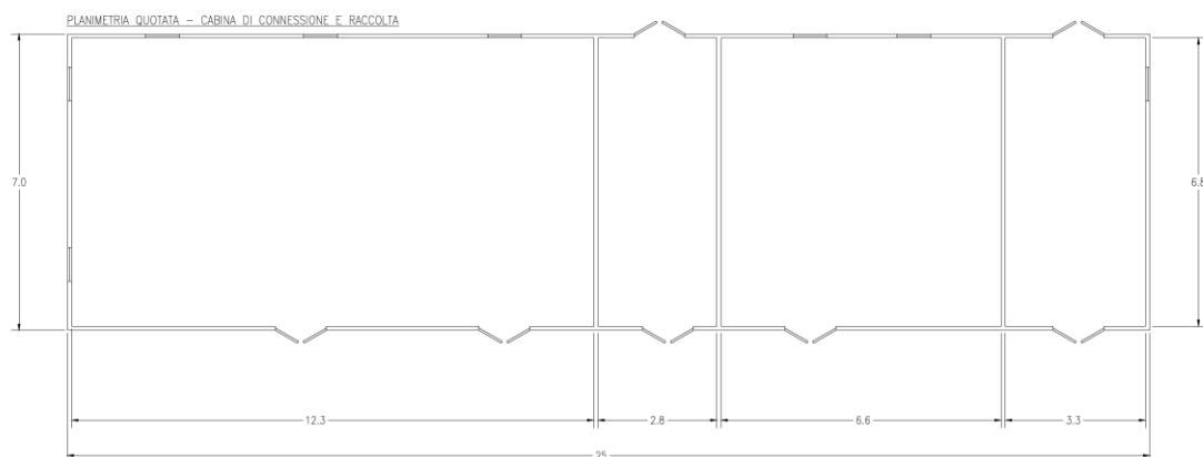
FIGURA 21: VISTE IN PIANTA E PROSPETTO CABINE DI RACCOLTA
