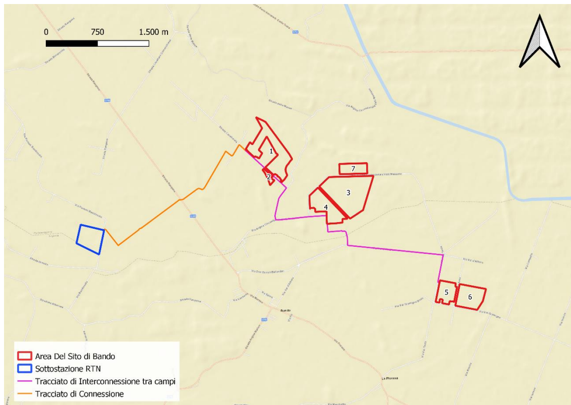
FIGURA 15: INQUADRAMENTO GEOGRAFICO DEL SITO CON CAVIDOTTO DI CONNESSIONE
