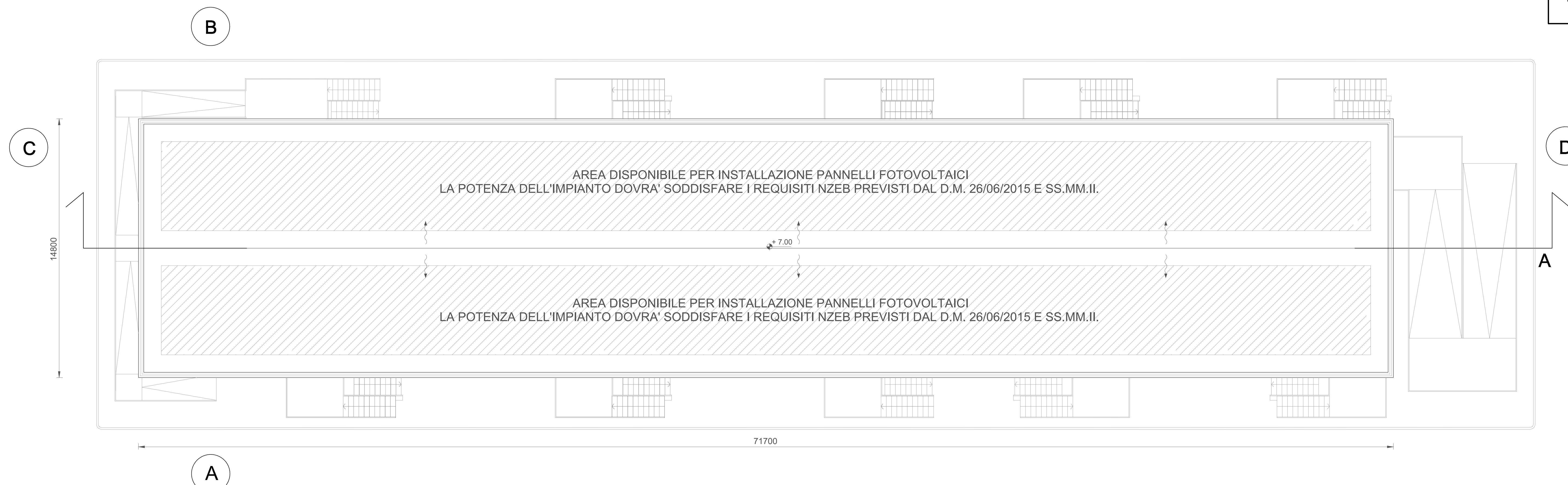
PIANTA COPERTURA
