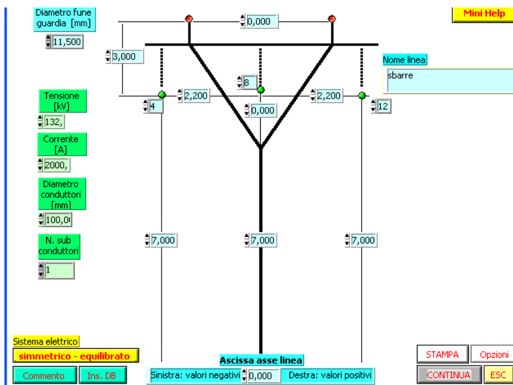
Figura 7: Linea AT con disposizione conduttori in piano assimilabile ad un sistema a sbarre a 150 kV
