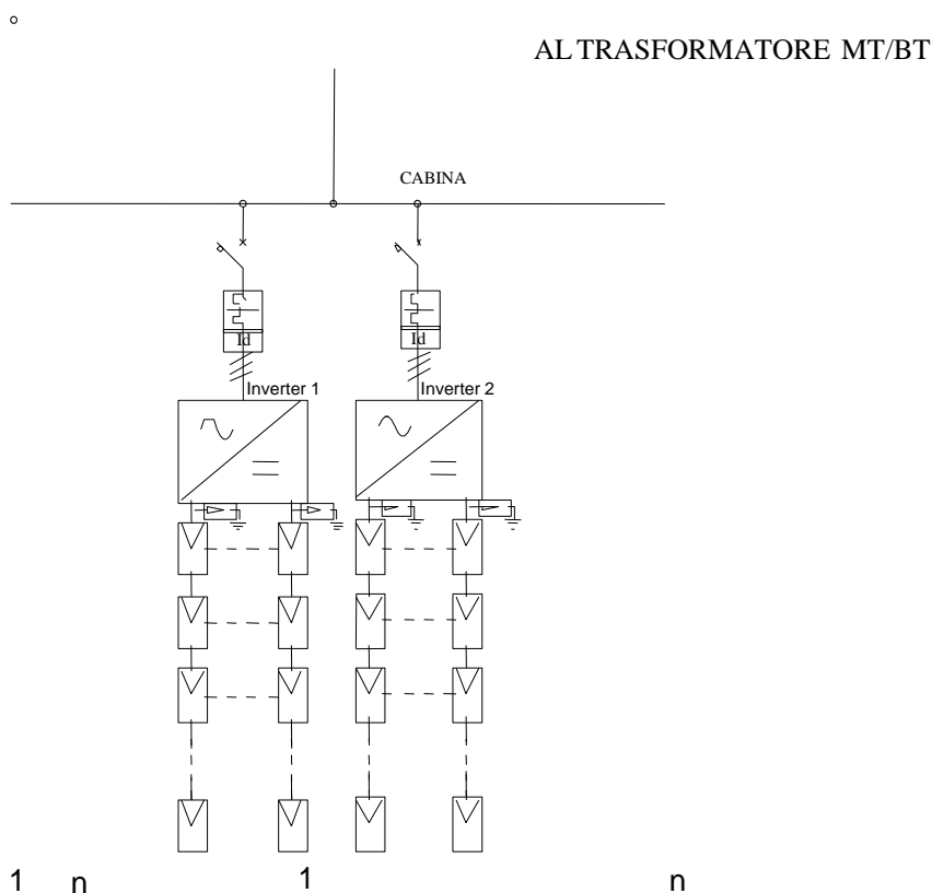
Figura 10: schema unifilare di principio dell'impianto fotovoltaico
