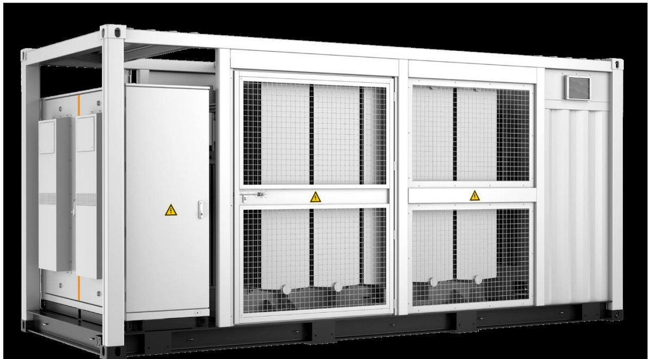
Figura 3 Foto trasformatore e relativo box di contenimento
