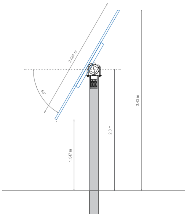
Struttura di supporto dei pannelli fotovoltaici
