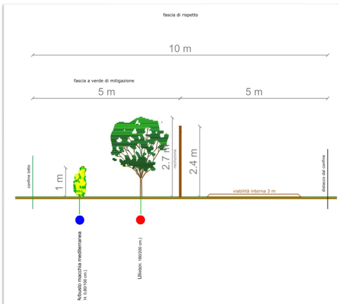
Stralcio sezione longitudinale opere mitigazione - TAVPROG007
