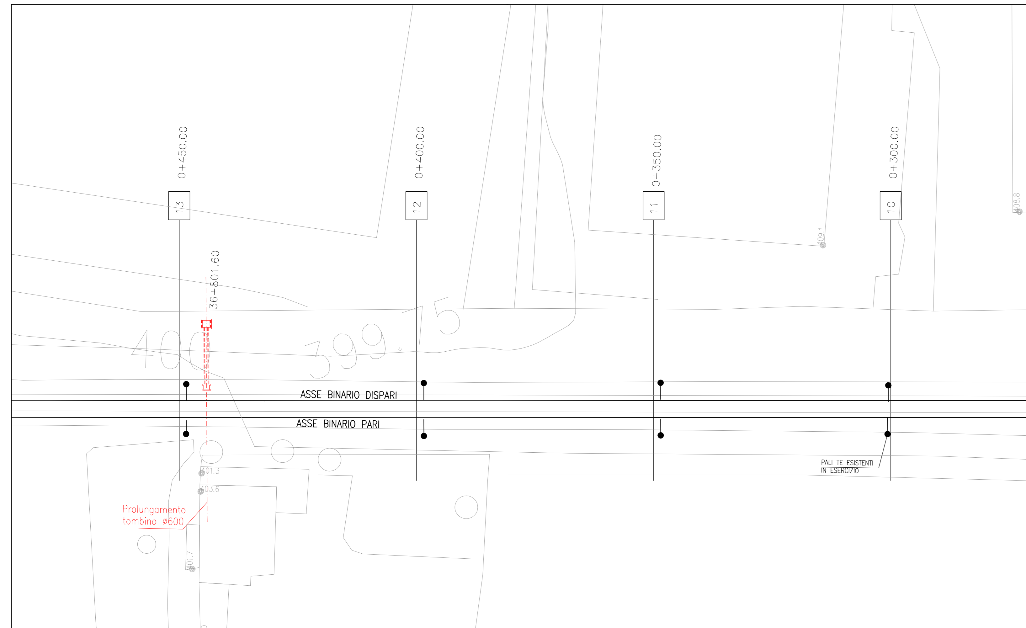
FASE 1 1:500
