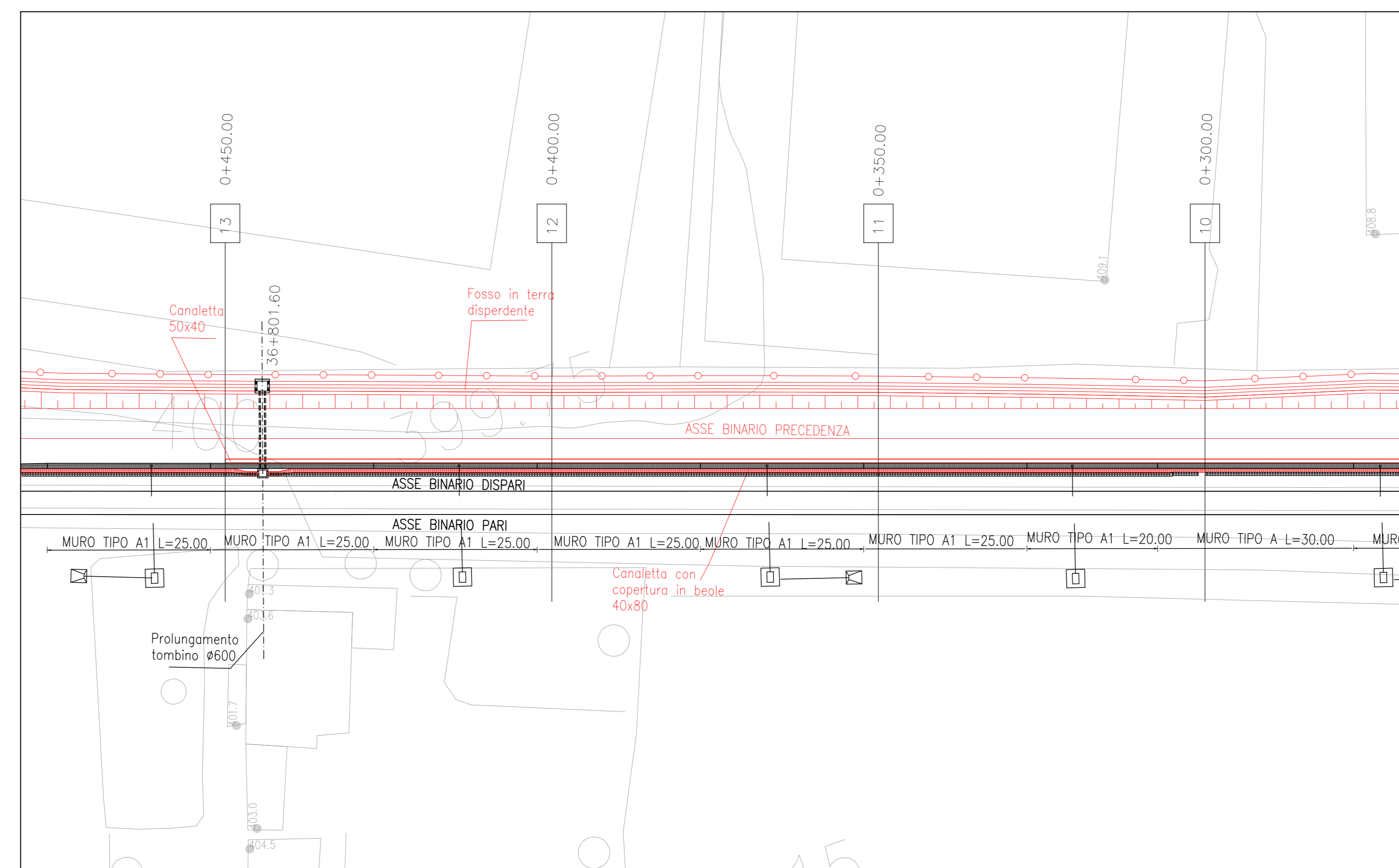
FASE 4 1:500
