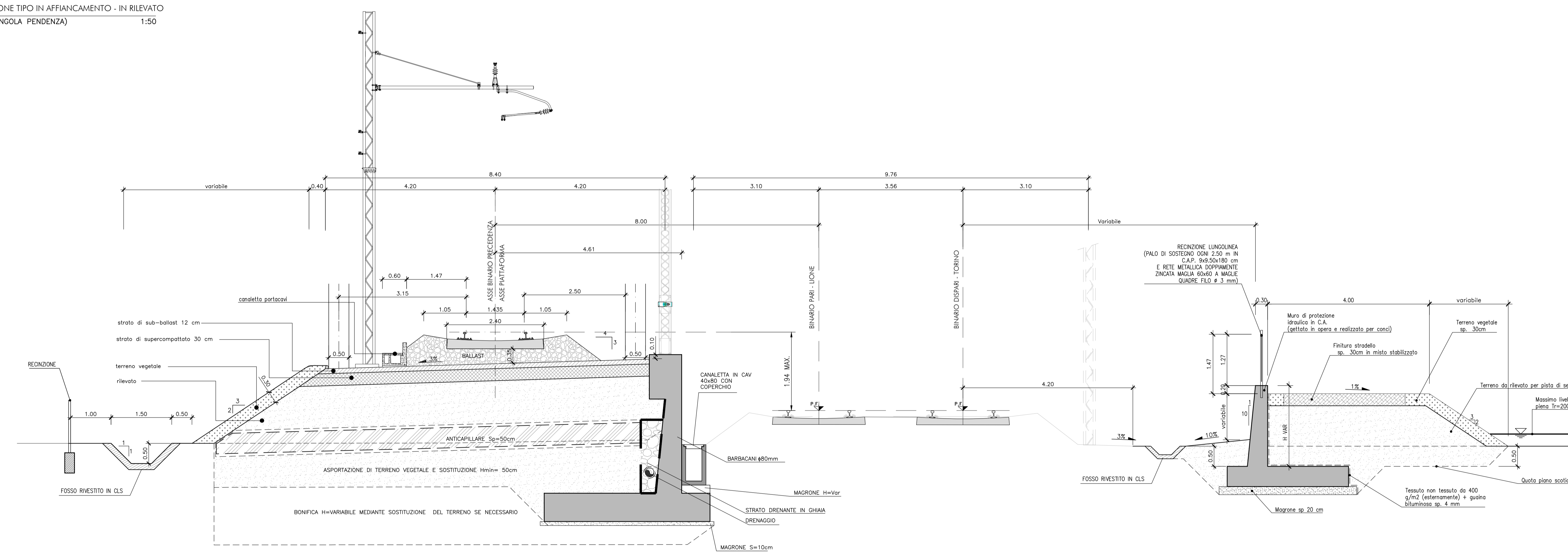
SEZIONE TIPO IN AFFIANCAMENTO - CON MURO DI SOSTEGNO 1:50
