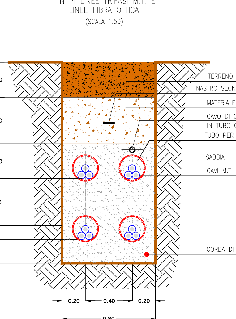
"SEZIONE TIPO 6-6" - TERRENO VEGETALE -
