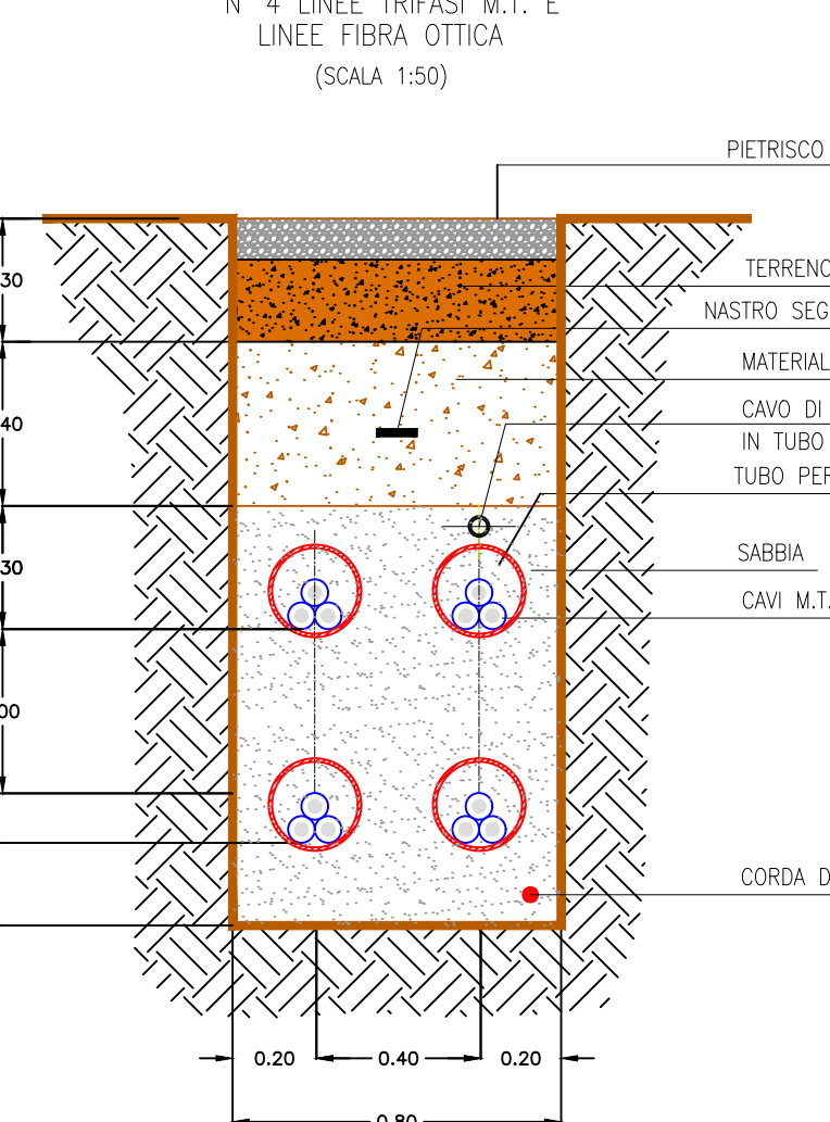
"SEZIONE TIPO 5-5" - STRADE NON ASFALTATE -
