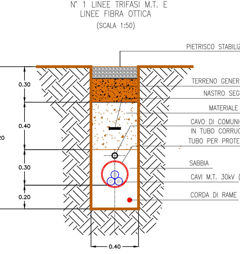
"SEZIONE TIPO 2-2" - STRADE NON ASFALTATE -
