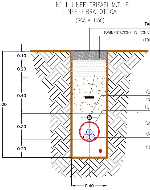
"SEZIONE TIPO 1-1" - STRADE ASFALTATE -
