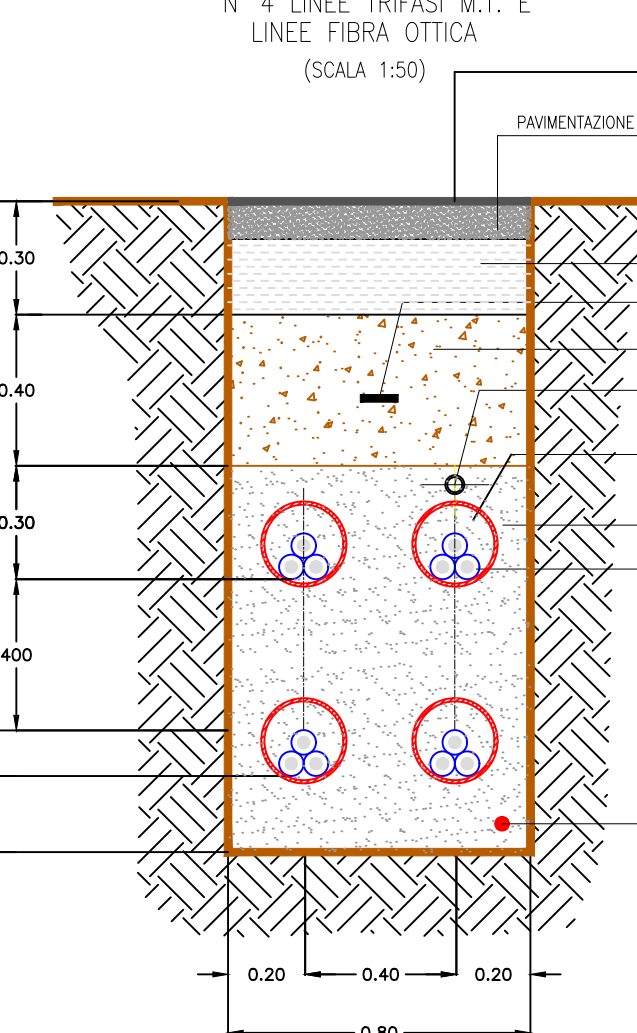
"SEZIONE TIPO 4-4" - STRADE ASFALTATE -
