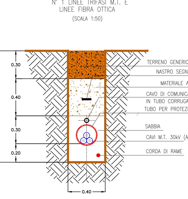
"SEZIONE TIPO 3-3" - TERRENO VEGETALE -
