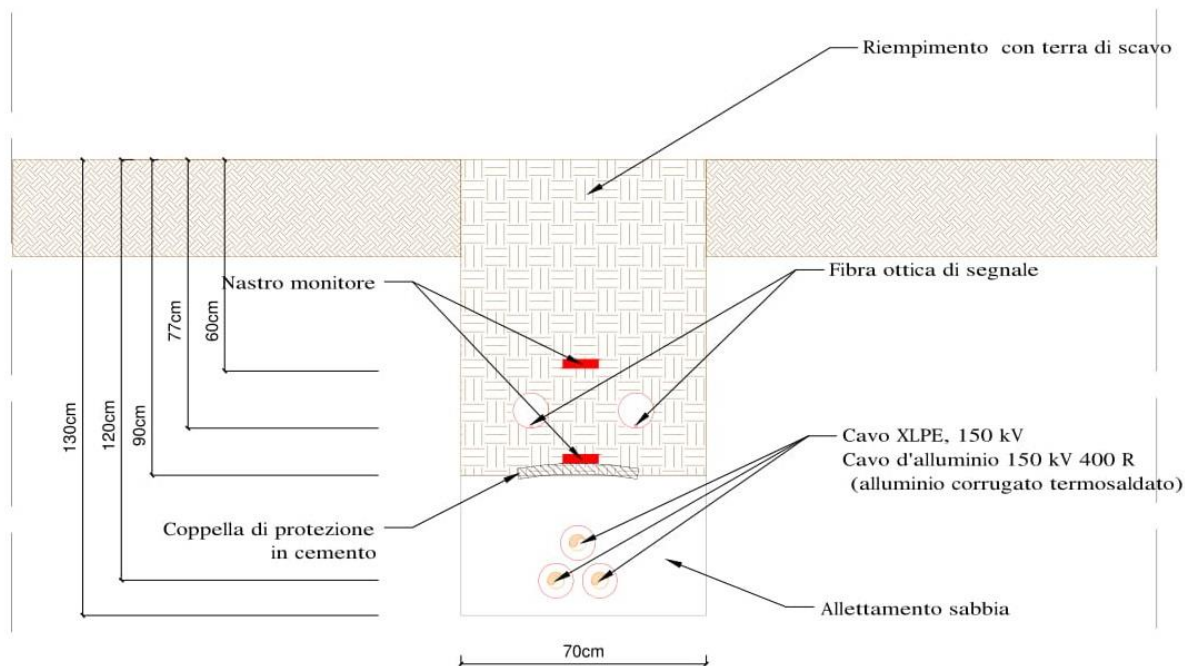
Figura 5.2: Sezione di Interramento Linea AT
