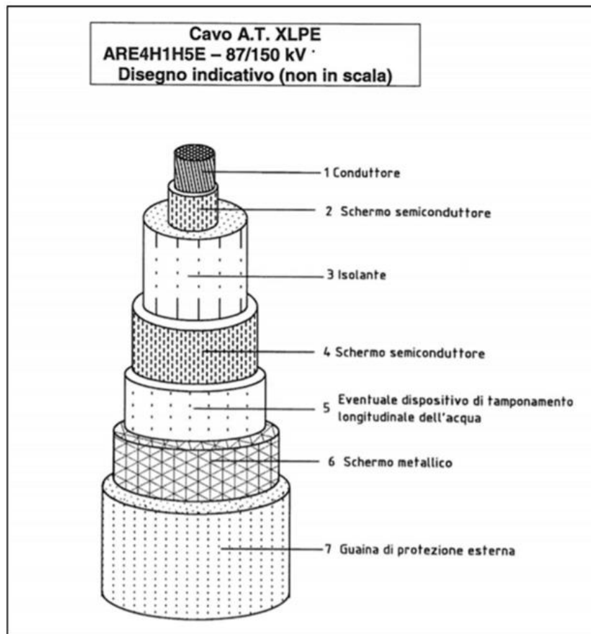
Figura 20: Sezione del cavo in AT
