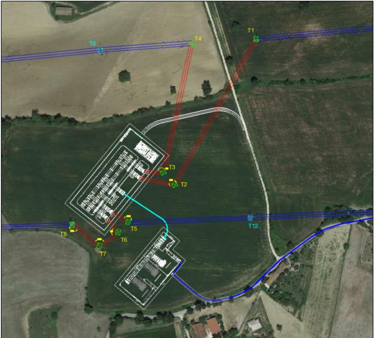
Figura 19: Inquadramento su ortofoto: stazione utente (bianco) collegata con la stazione elettrica di smistamento a 132 kV da realizzare in località di "Arcofiato", il cavidotto in AT di collegamento condiviso (in ciano)
