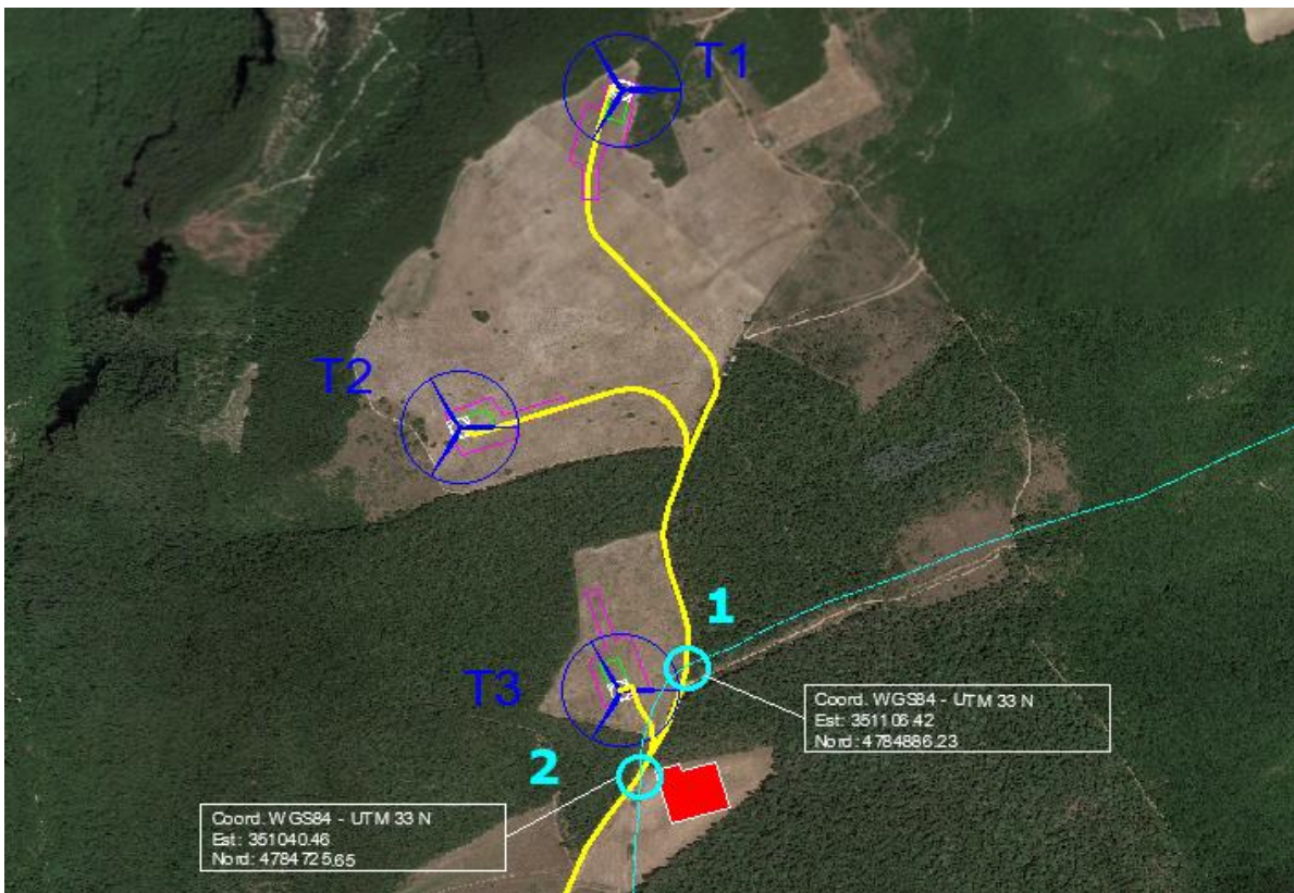
Figura 12: Riquadro 1 di Figura 13 in cui è visibile l'attraversamento del metanodotto interrato in due punti (N°1,2).
