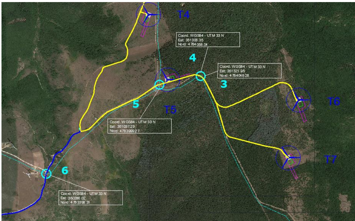
Figura 13: Riquadro 2 di Figura 13 in cui è visibile l'attraversamento dei metanodotti interrati (ciano) in 4 punti (N°3-6).
