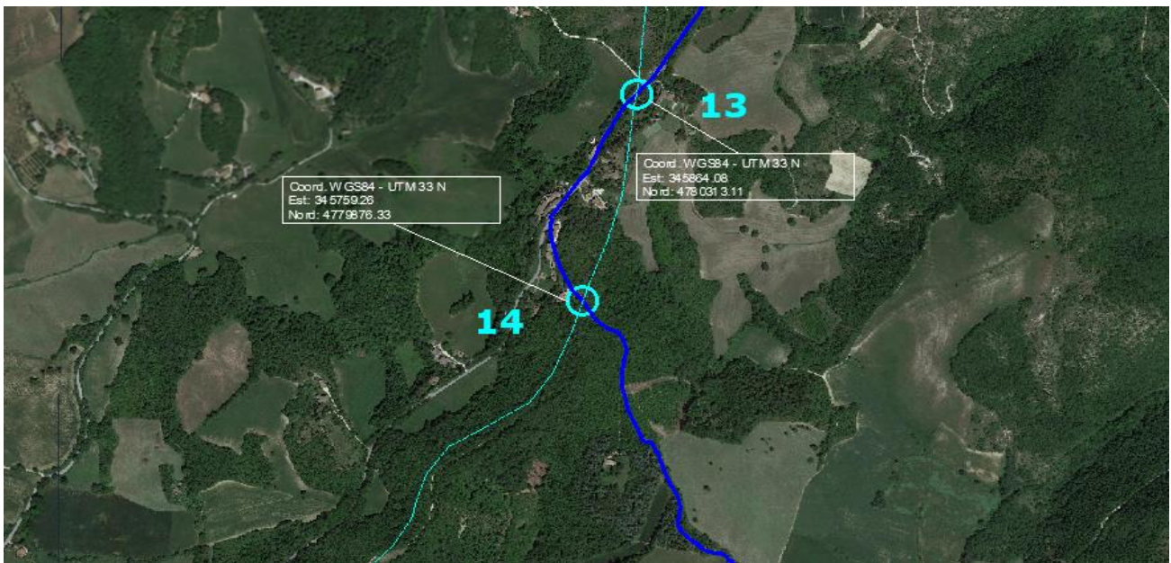
Figura 16: Riquadro 5 di Figura 13 in cui è visibile l'attraversamento dei metanodotti interrati (ciano) in due punti (N°13,14).
