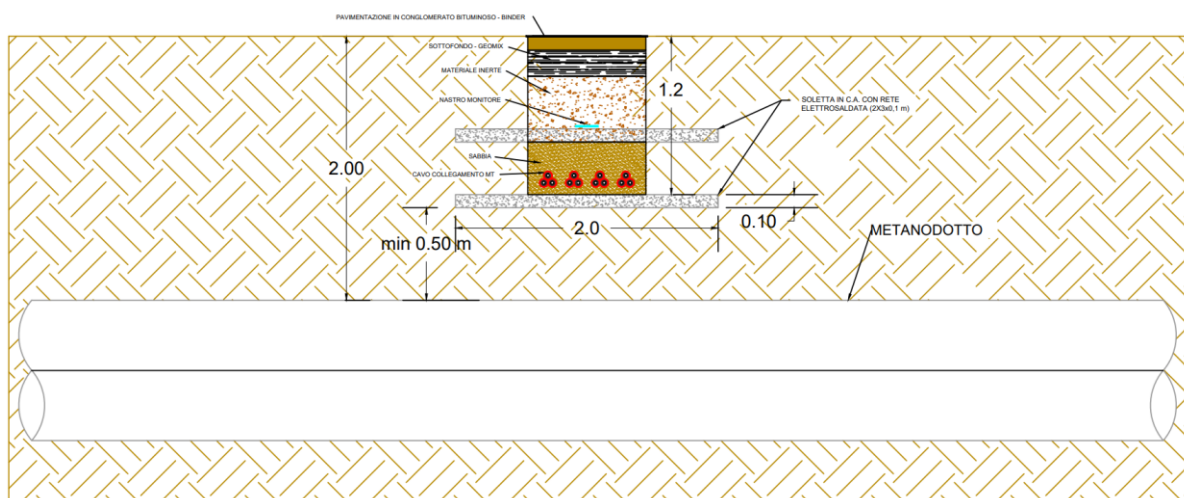
Figura 3: Tipico attraversamento dei metanodotti
