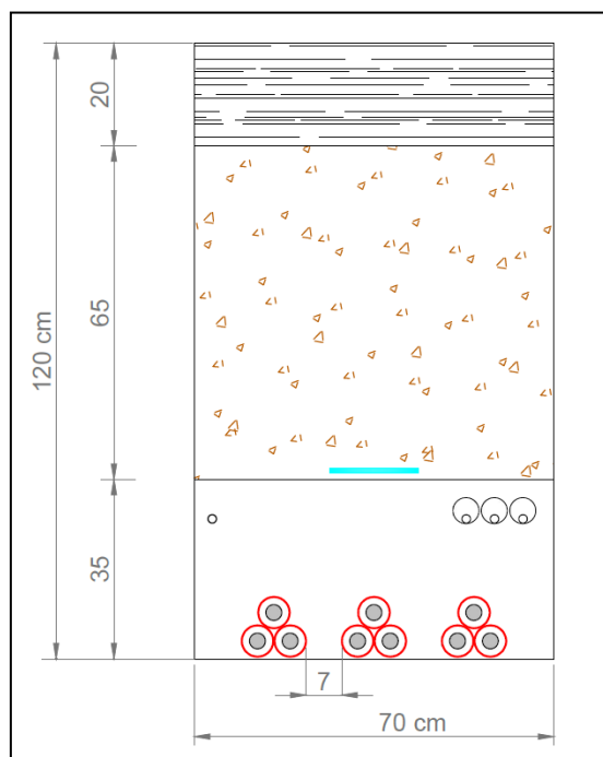
Figura 8 – Sezione tipo del cavidotto interrato MT composto da n.3 terne di cavi su strada sterrata
