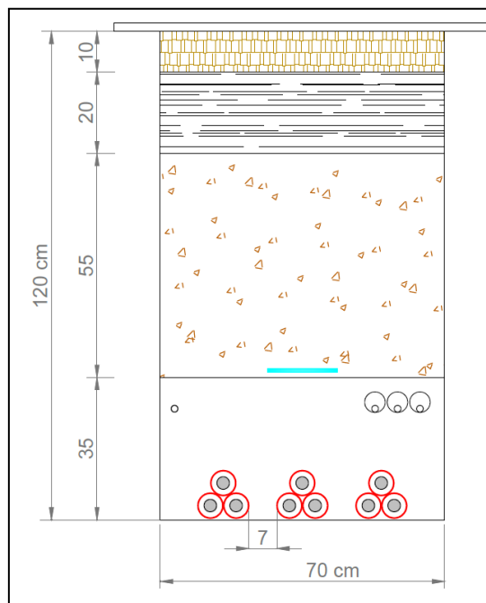
Figura 7 – Sezione tipo del cavidotto interrato MT composto da n.3 terne di cavi su strada asfaltata
