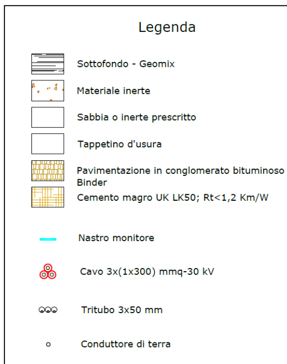
Figura 10: Materiali di riempimento per tipologia di scavo
