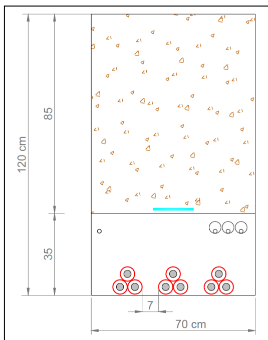
Figura 9 – Sezione tipo del cavidotto interrato MT composto da n.3 terne di cavi su terreno
