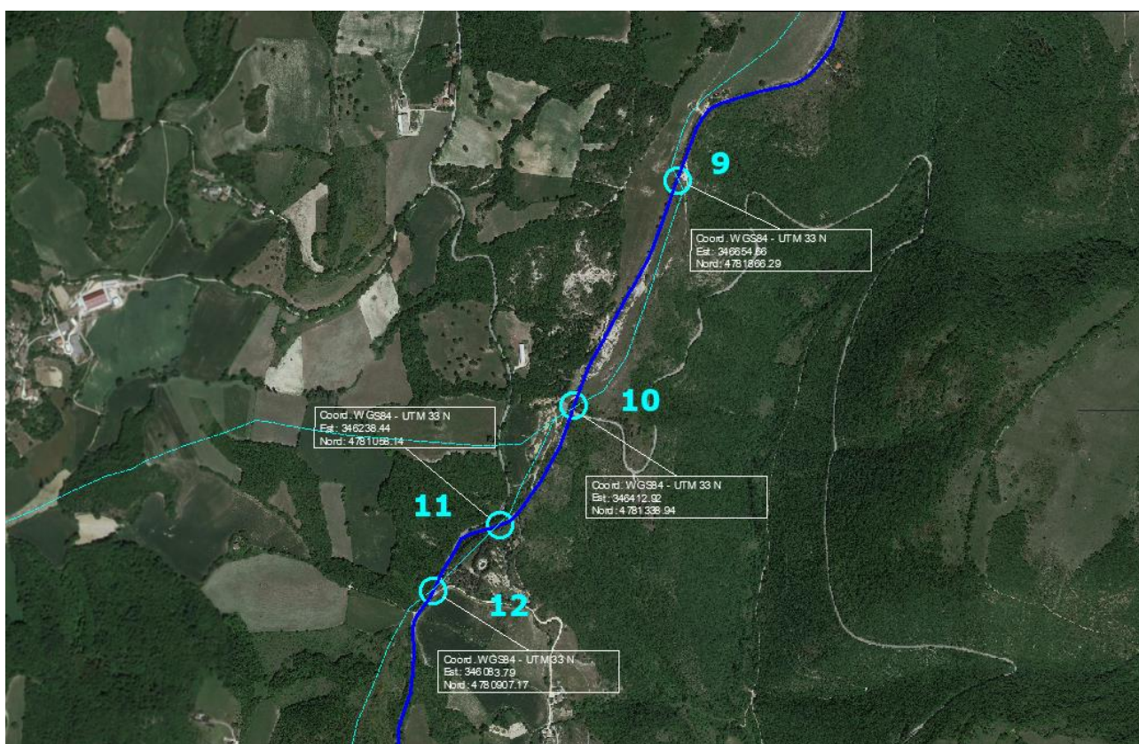
Figura 15: Riquadro 4 di Figura 13 in cui è visibile l'attraversamento dei metanodotti interrati (ciano) in quattro punti (N° 9-12).
