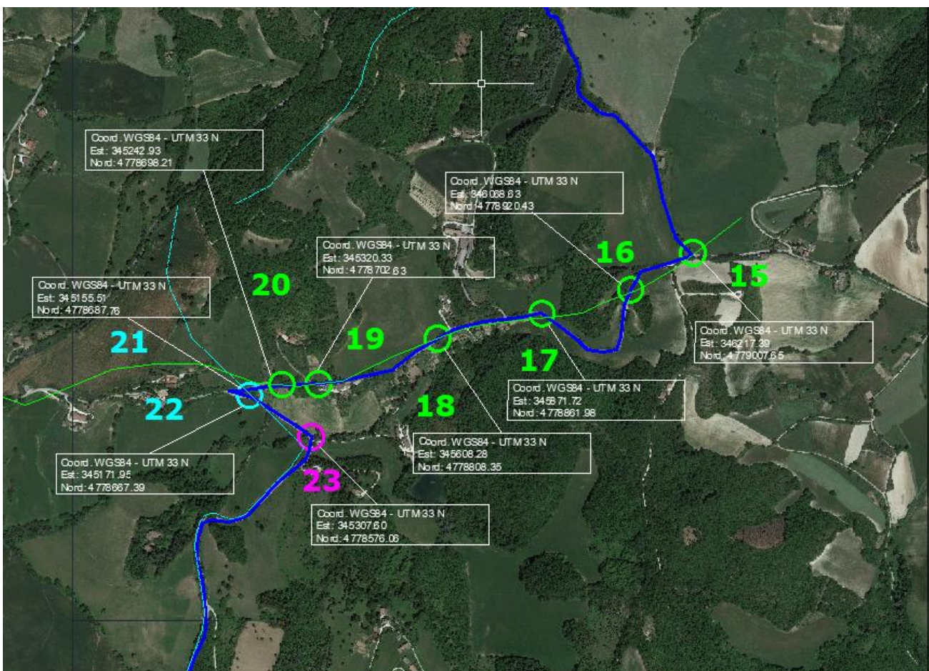
Figura 17: Riquadro 6 di Figura 13 in cui è visibile l'attraversamento un acquedotto interrato (verde) in 6 punti (N° 15-20), l'attraversamento de un metanodotto interrato in 2 punti (N°21-
