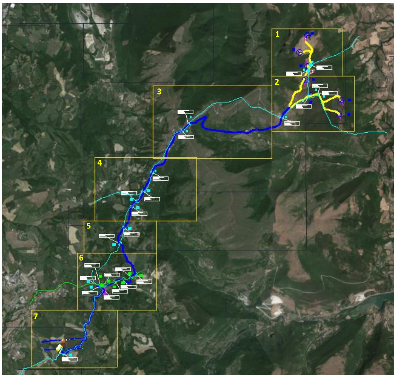
Figura 11: Inquadramento su ortofoto: impianto eolico, cavidotti in MT (in giallo e in blu) e attraversamento delle interferenze.
