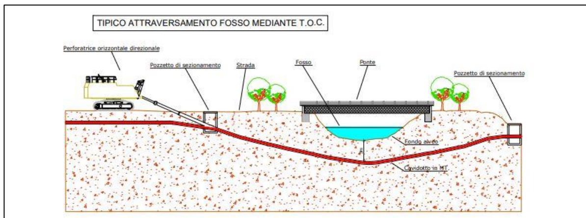
Figura 12: Attraversamento tipo mediante tecnica TOC dei fossi
