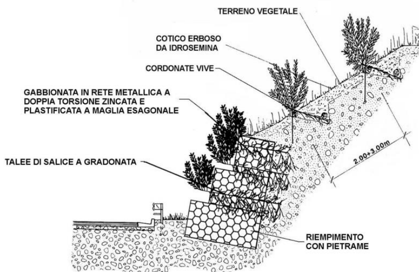
Figura 5: Esempio di inserimento di gabbionate rinverdate
