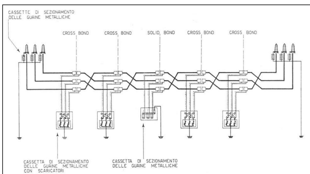
Figura 19: Tipico collegamento "cross bonding" per un cavo in AT
