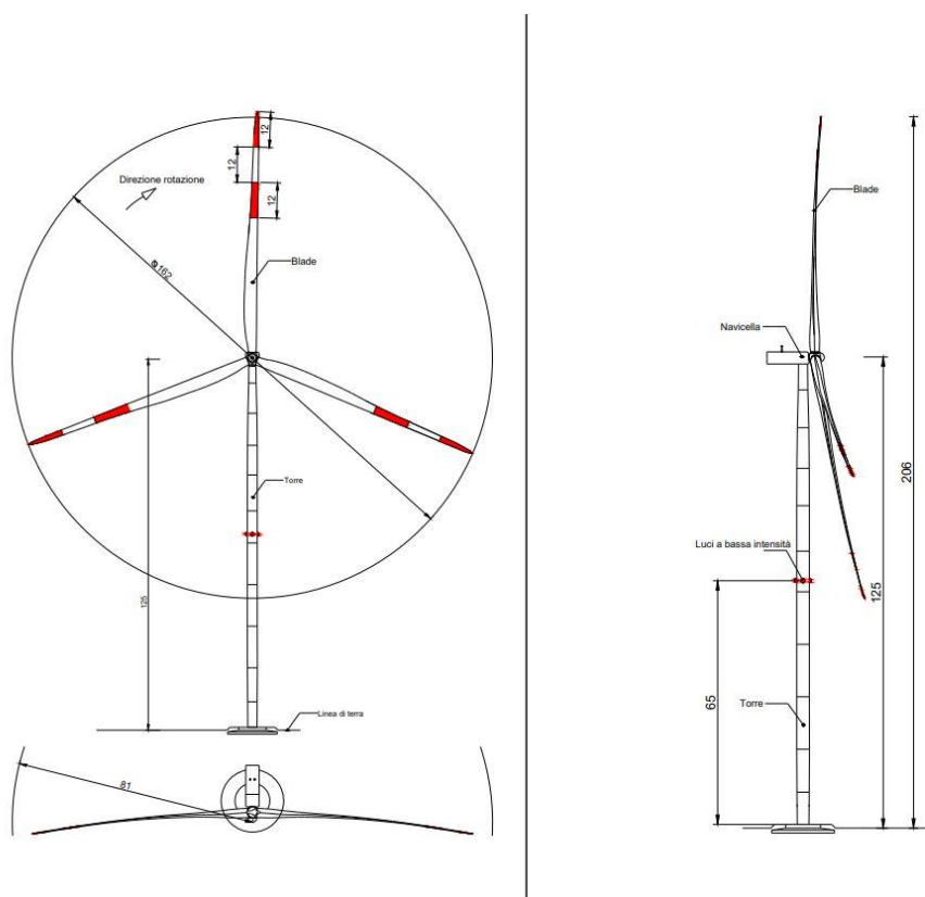
Figura 8: Vista frontale e laterale dell'aerogeneratore V162 – 6,0
