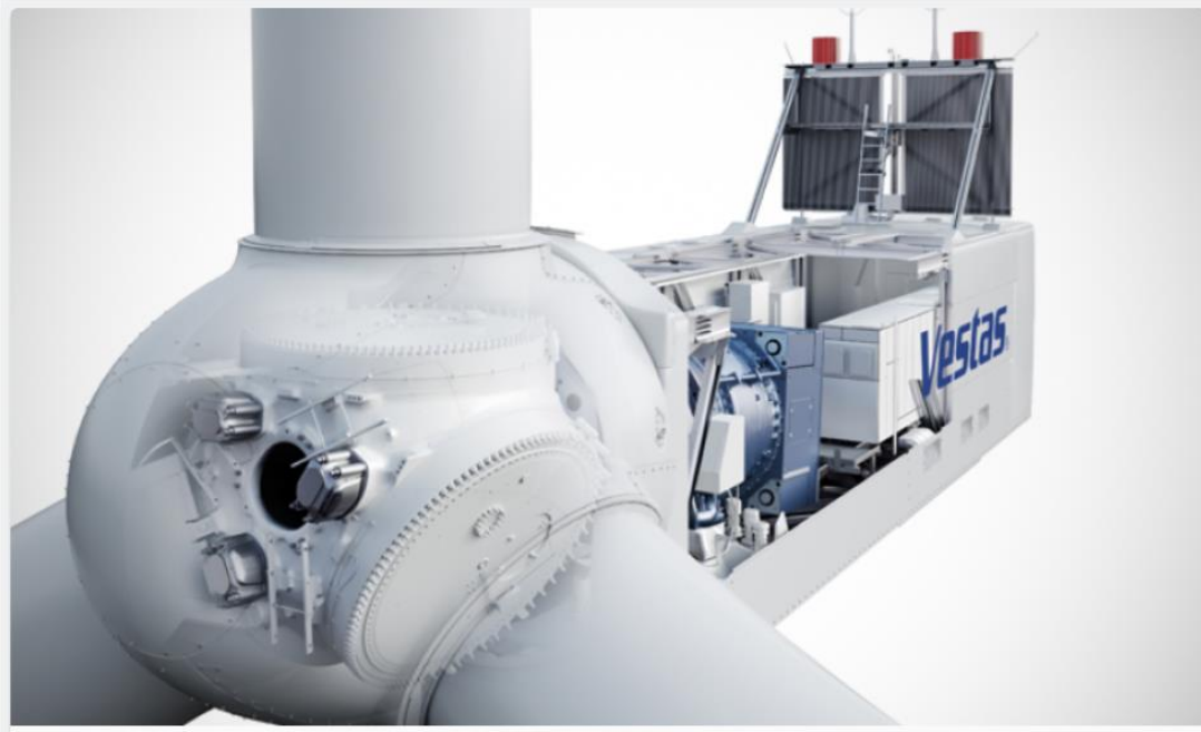
Figura 5 - Spaccato aerogeneratore tipo, modello V162
