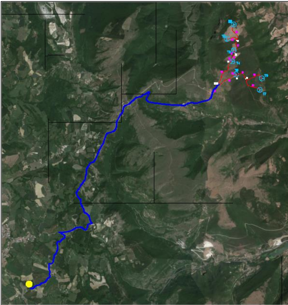
Figura 2 –Stralcio dell’ ortofoto con indicazione delle aree d’ impianto, del cavidotto di connessione, della SU e della SE (area in giallo)
