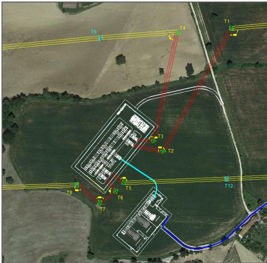
Figura 18 –Stralcio su ortofoto della posizione della SU, del cavidotto in AT (in ciano), della Stazione SE e di raccordi (in rosso)
