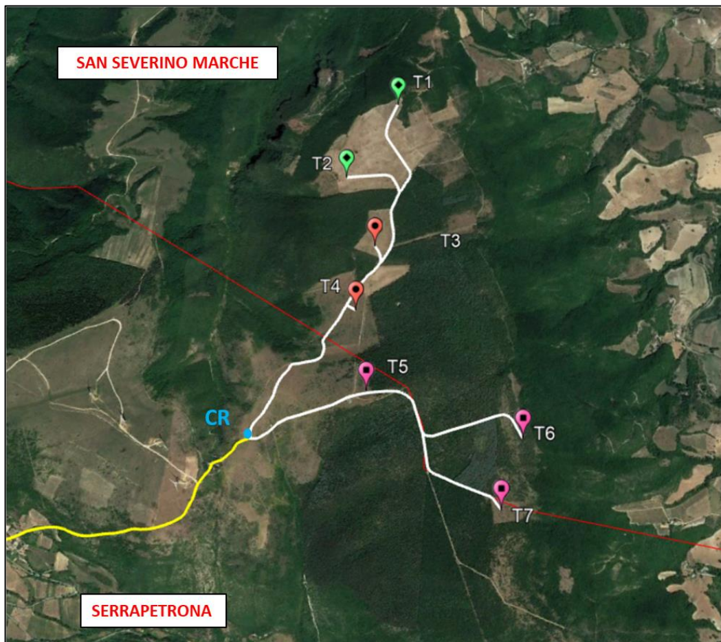
Figura 1 - Stralcio dell' ortofoto con indicazione delle posizione delle trubine
