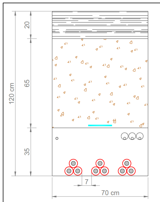
Figura 11 – Sezione tipo del cavidotto interrato MT composto da n.3 terne di cavi su strada sterrata
