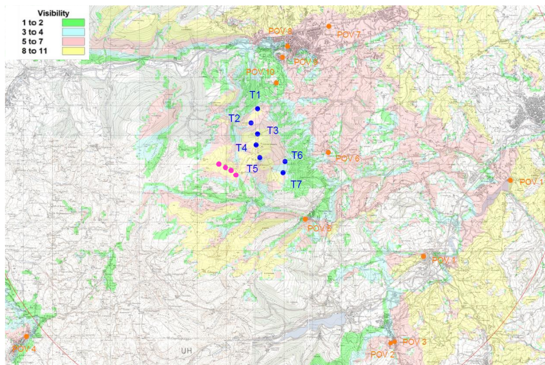
Figura 6 – Stralcio di cartografia IGM 1:25000 con indicazione delle zone di visibilità degli aerogeneratori, in progetto (in blu) ed esistenti (in fuxia), e dei ricettori (in arancione) – caso 1.
