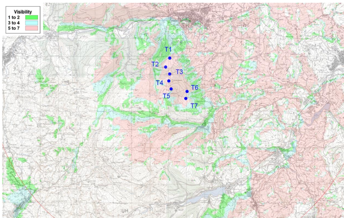
Figura 3: Stralcio di cartografia IGM 1:25.000 con indicazione delle zone di visibilità degli aerogeneratori in progetto – Impianto in progetto - caso 2.
