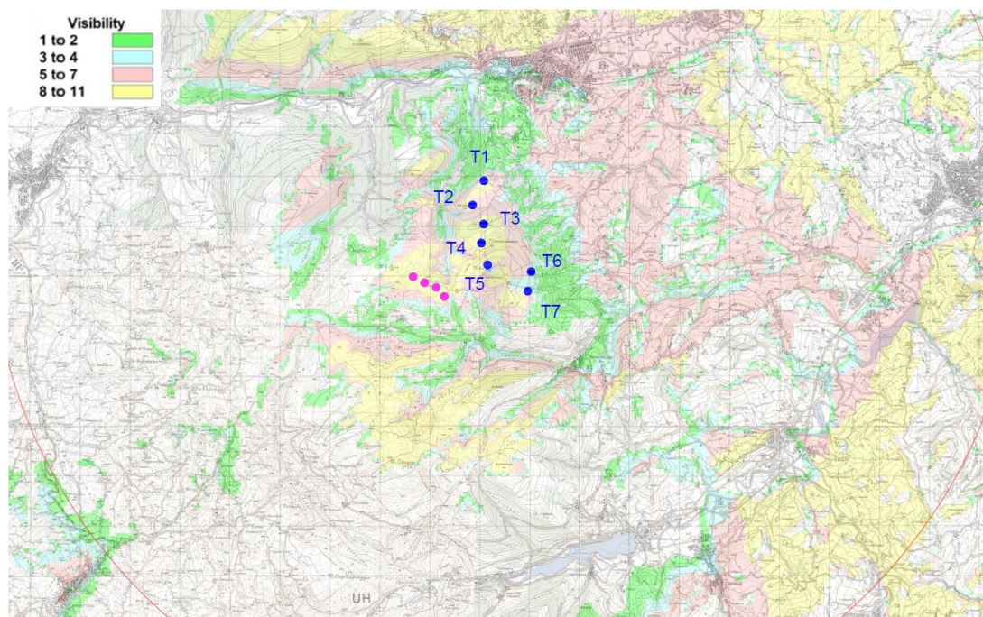
Figura 4: Stralcio di cartografia IGM 1:25000 con indicazione delle zone di visibilità degli aerogeneratori, progetto (in blu) ed esistenti (in fuxia) – Impianto in progetto con impianto esistente - caso 1.
