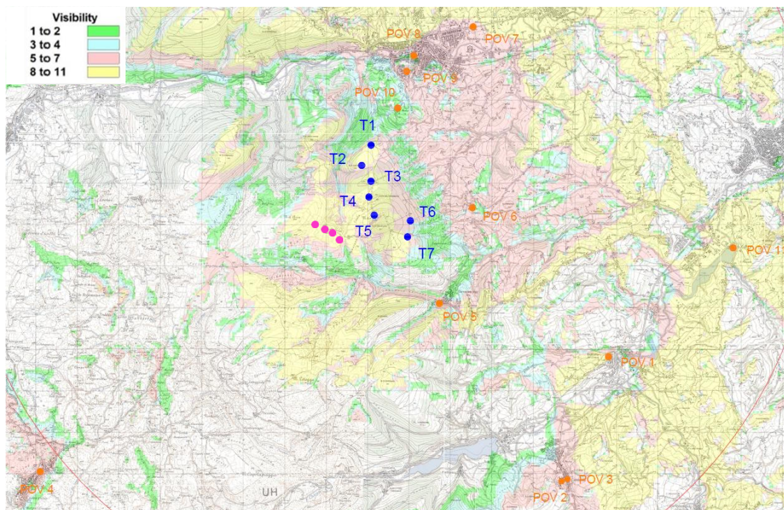
Figura 7 – Stralcio di cartografia IGM 1:25000 con indicazione delle di visibilità degli aerogeneratori, in progetto (in blu) ed esistenti (in fuxia), e dei ricettori (in arancione) – caso 2.
