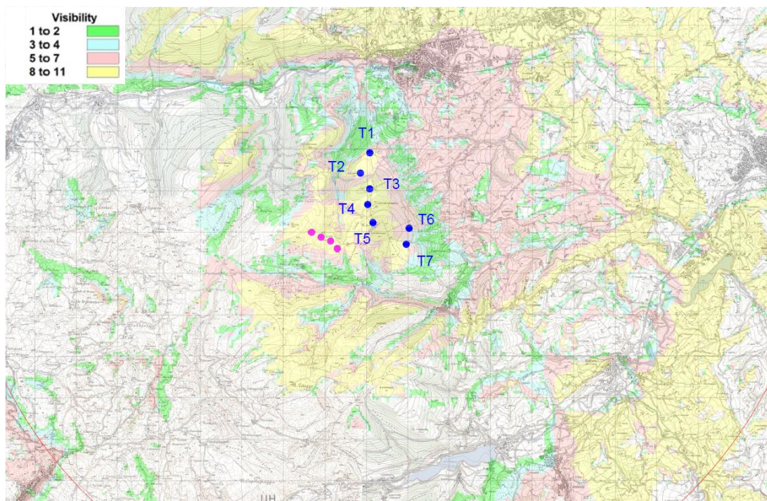
Figura 5: Stralcio di cartografia IGM 1:25000 con indicazione delle zone di visibilità degli aerogeneratori, in progetto (in blu) ed esistenti (in fuxia) – Impianto in progetto con impianto esistente - caso 2.
