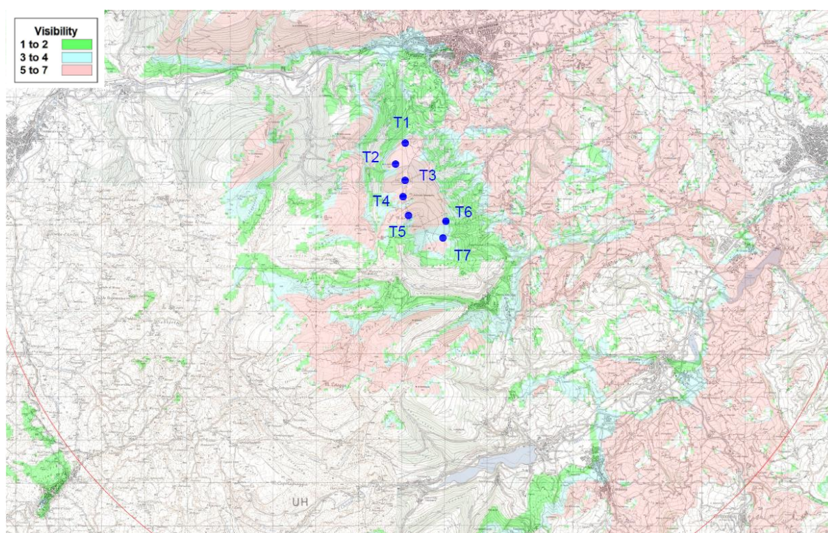
Figura 2: Stralcio di cartografia IGM 1:25000 con indicazione delle zone di visibilità degli aerogeneratori in progetto – Impianto in progetto - caso 1.
