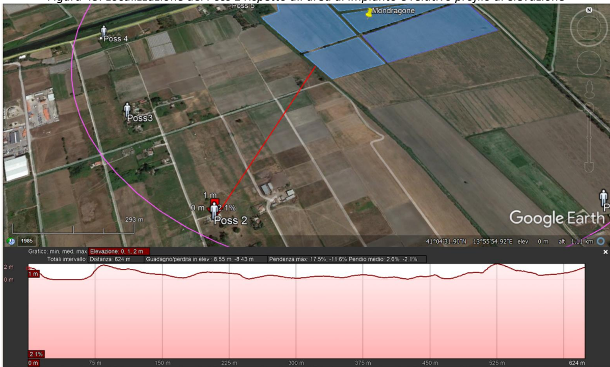
Figura 46. Localizzazione del Poss 2 rispetto all'area di impianto e relativo profilo di elevazione
