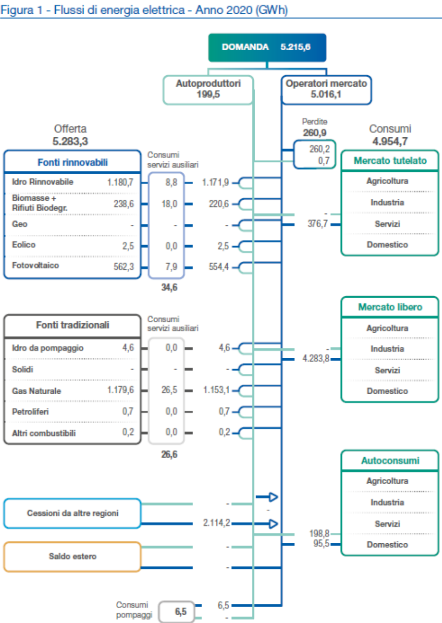
Figura 29 - flussi di energia elettrica, Umbria
