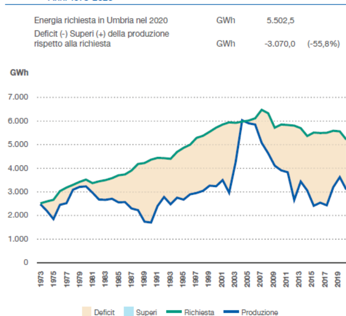
Figura 4 – Serie storica superi (+) e deficit (-) della produzione rispetto alla richiesta, Anni 1973-2020
