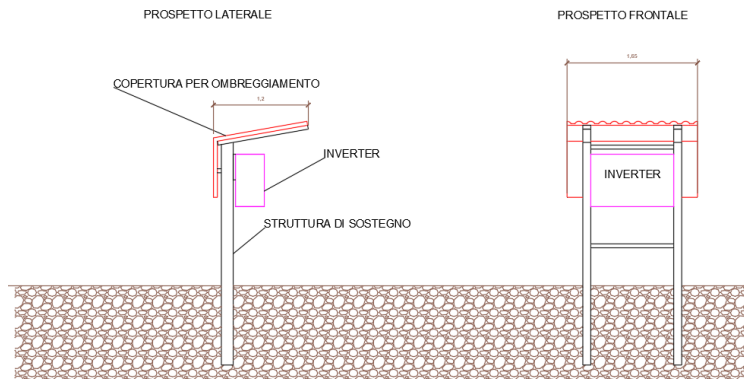
Fig. 12 - Tipico struttura supporto inverter
