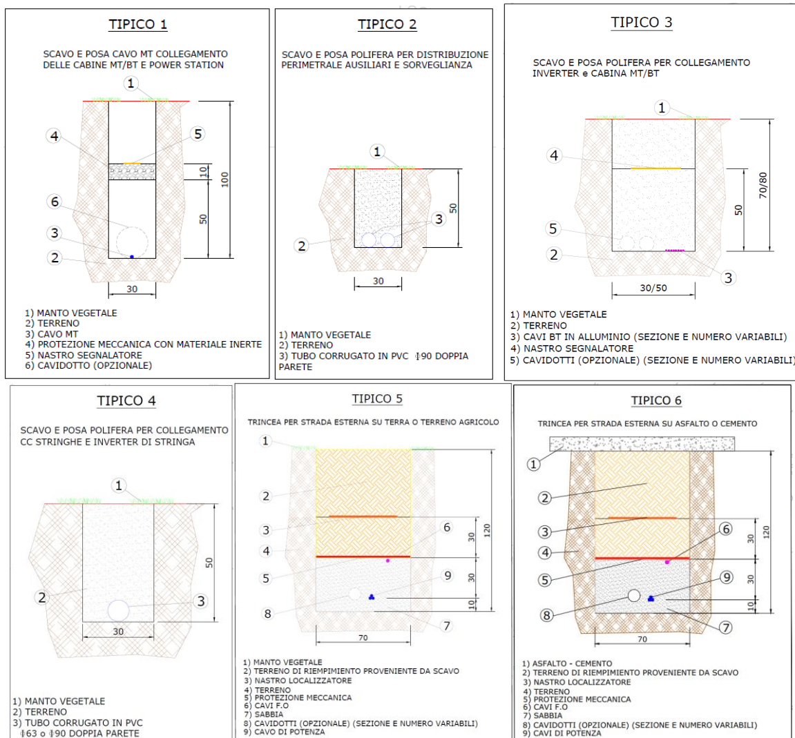
Fig. 20 – Tipici scavi e posa cavi
