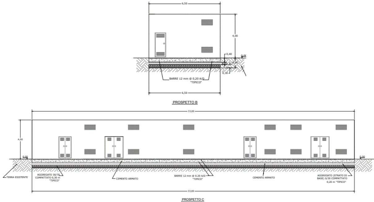
Fig. 22 - Cabina di ricezione
