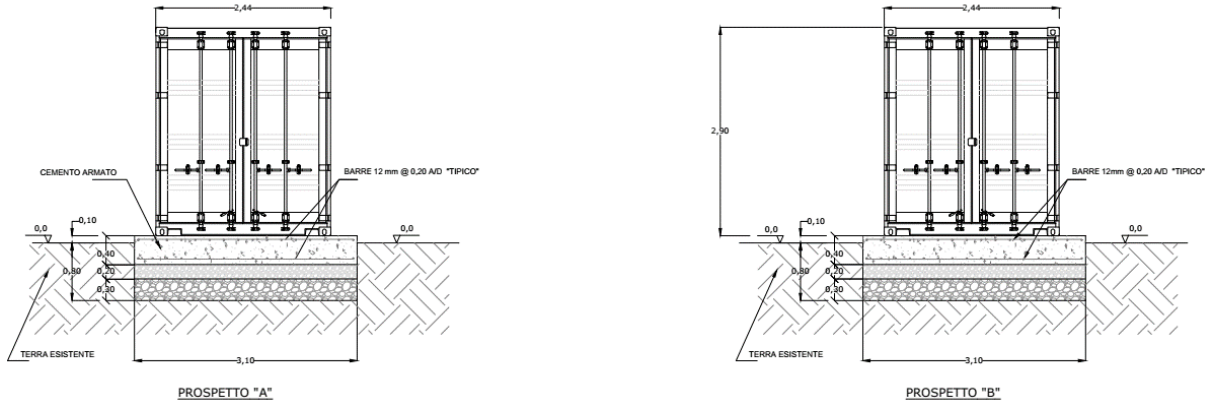
Fig. 21 - Cabina di trasformazione BT/MT
