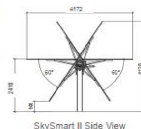
Fig. 11 – Dimensioni, specifiche tecniche e prestazionali Inseguitori solari (tracker)
