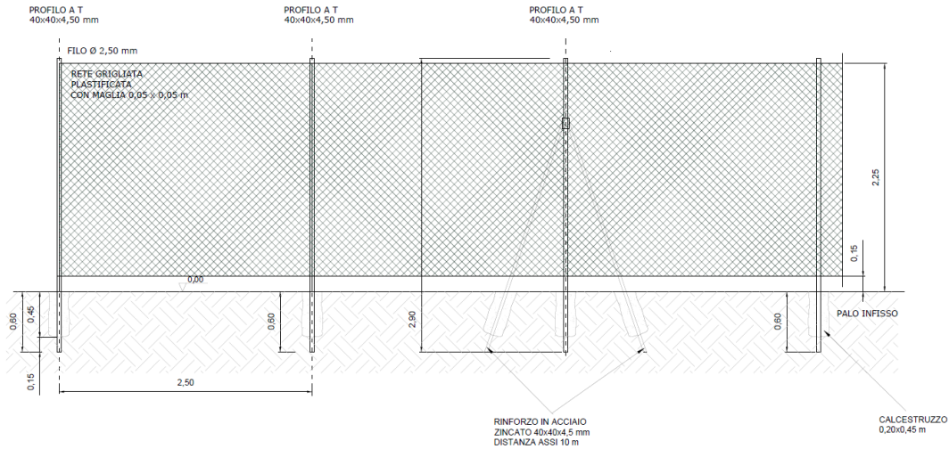
Fig. 17 – Recinzione perimetrale
