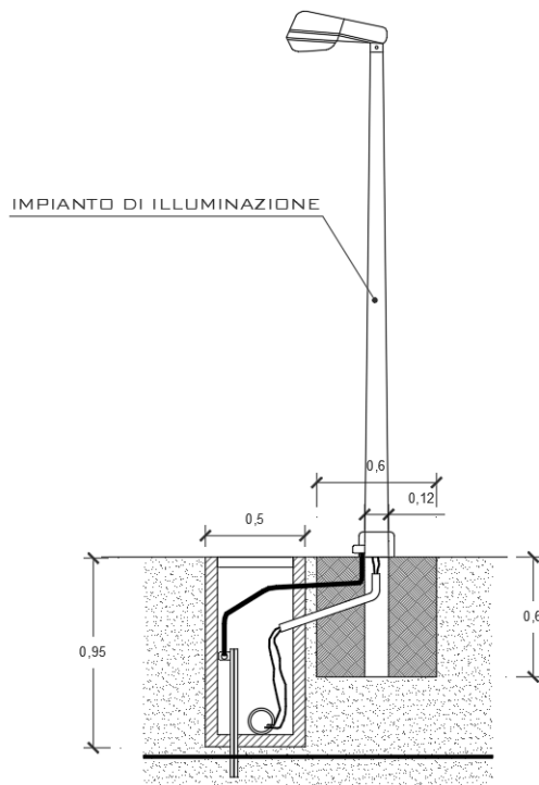
Fig. 25 – Sistema di illuminazione
