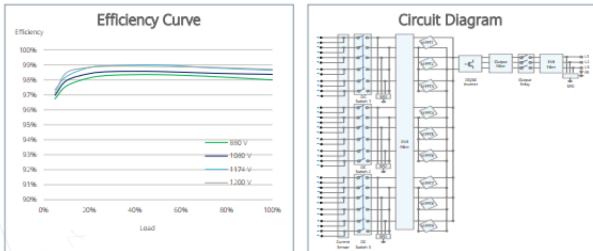
Fig. 15 - Dimensioni, specifiche tecniche e prestazionali dell'inverter
