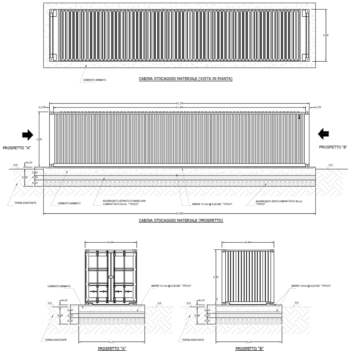
Fig. 23 - Cabina stoccaggio materiale
