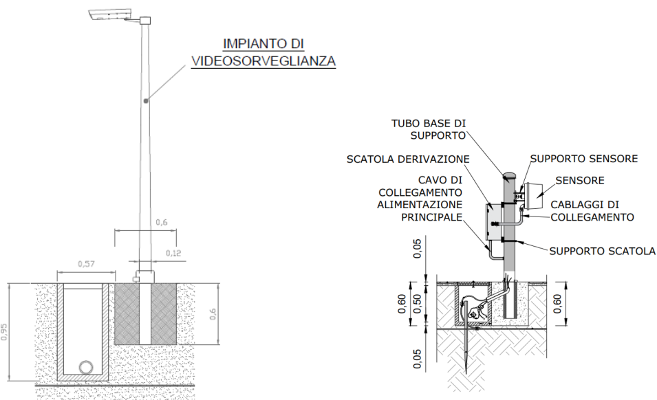
Fig. 19 – Sistema antintrusione
