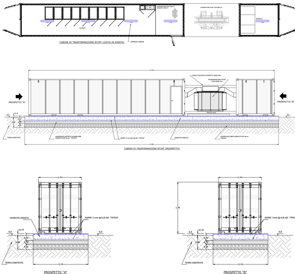
Fig.13 – Cabina di trasformazione BT/MT
