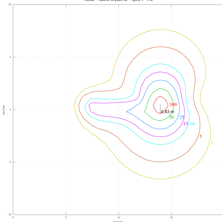
Cabina - calcolo su piano xz - quote Y=-1 m
