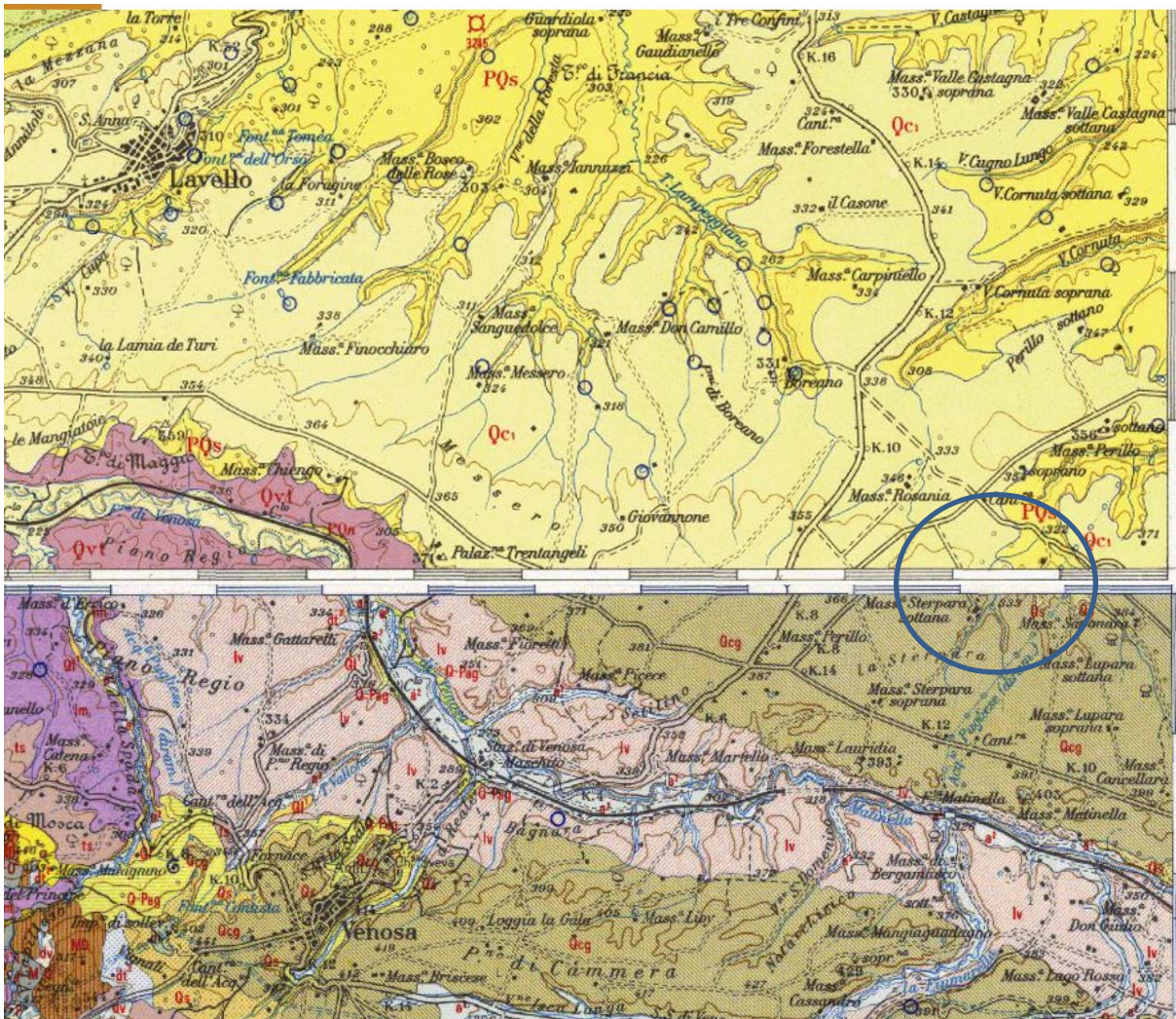
STRALCIO CARTA GEOLOGICA F° 175 E 187
