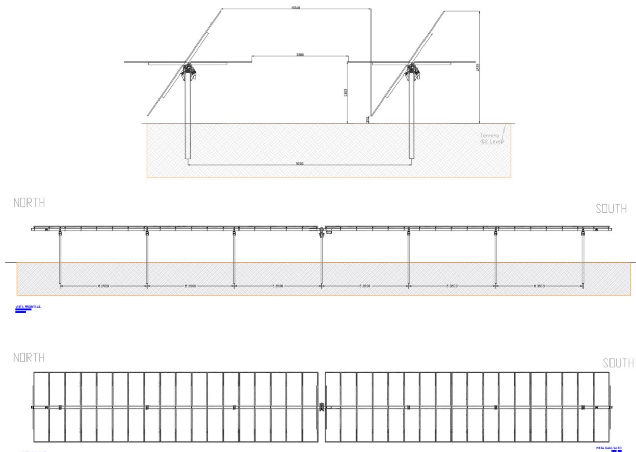
Viste del tracker: laterali, frontale e dall'alto
